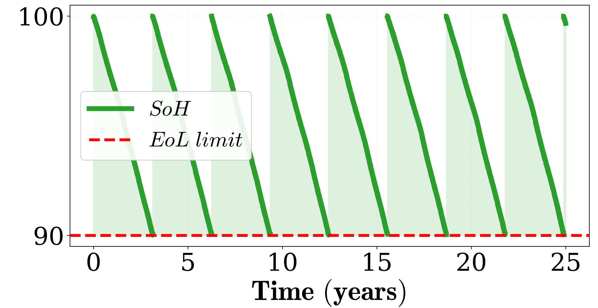
PEMWE Degradation
