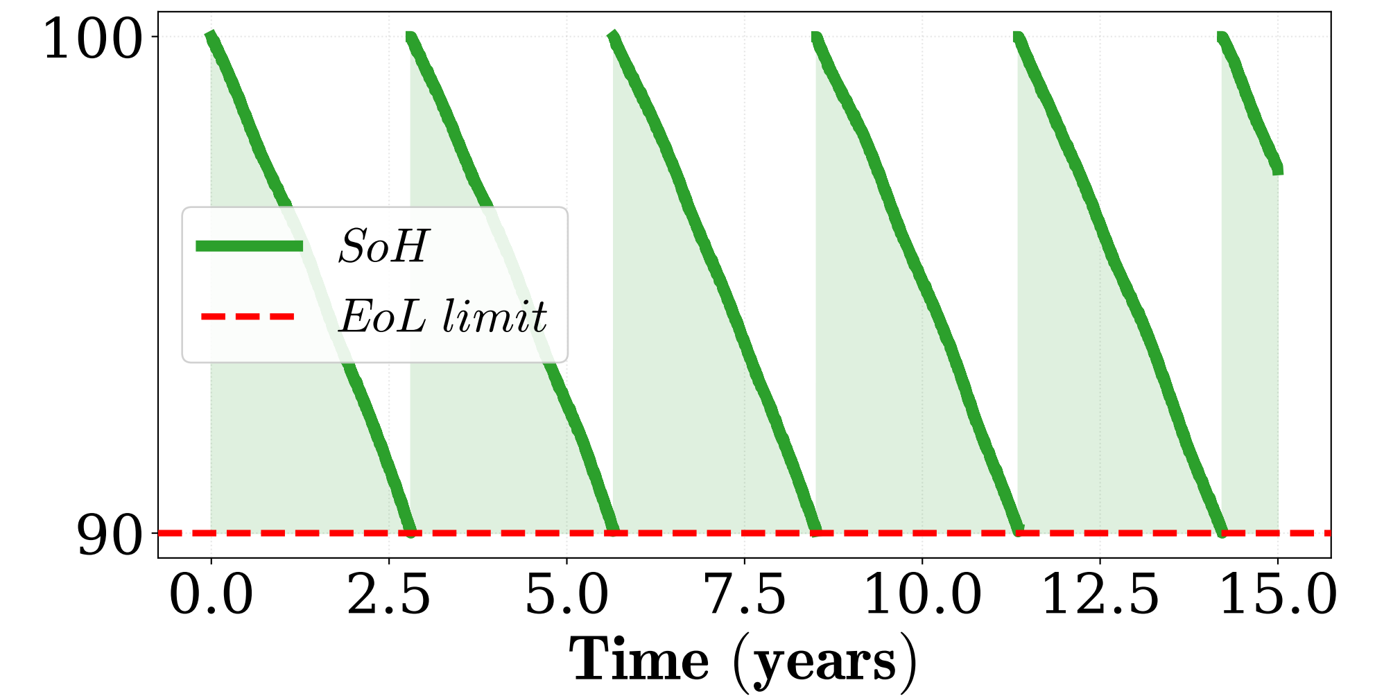
PEMWE Degradation
