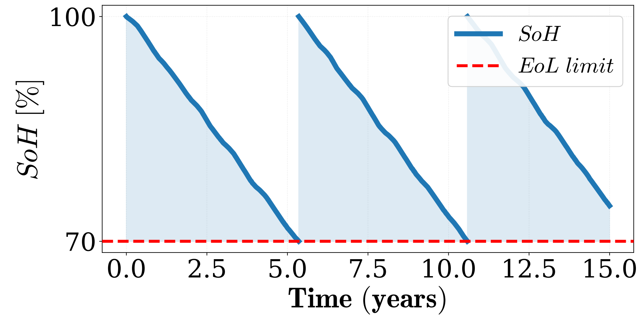
PEMFC Degradation
