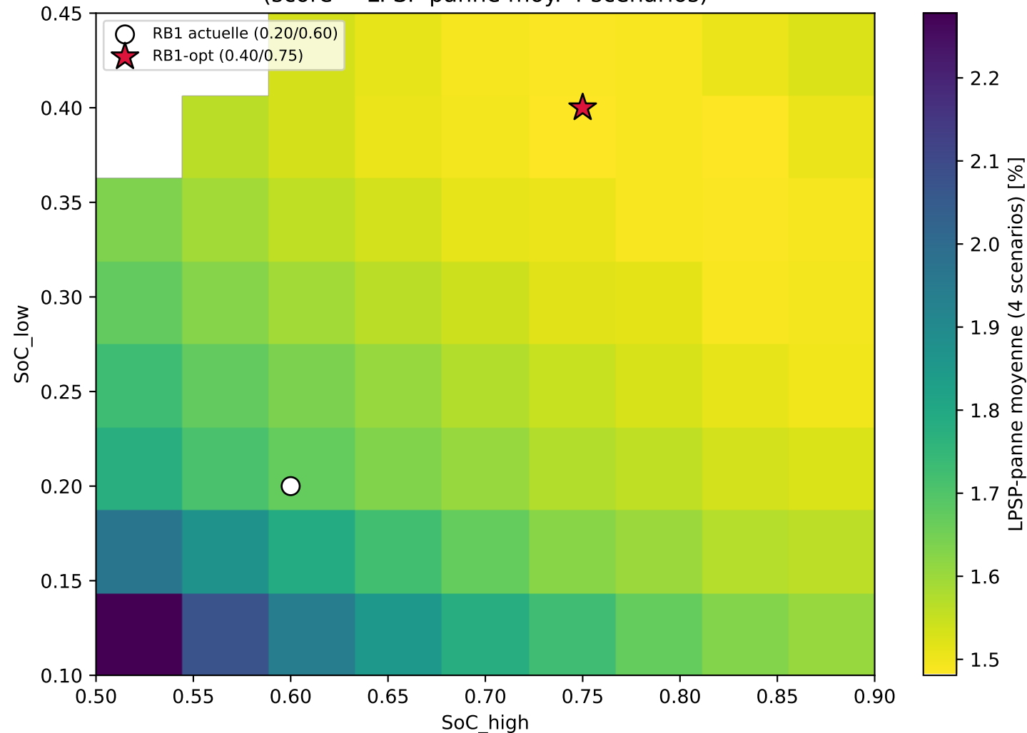
Sweep RB1 -- robustesse sous defaillance (score = LPSP-panne moy. 4 scenarios)
