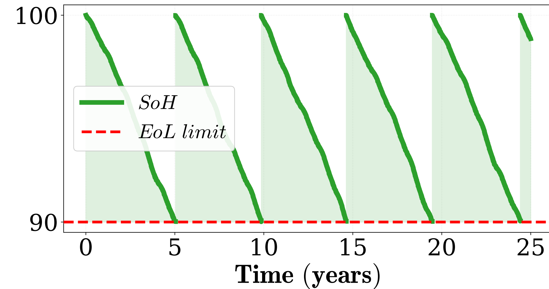
PEMWE Degradation
