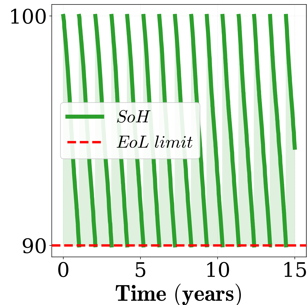
PEMWE Degradation
