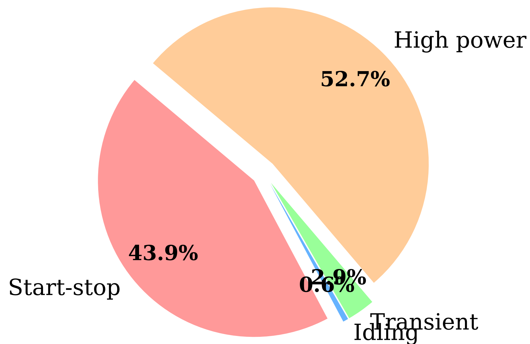
PEMFC Degradation
