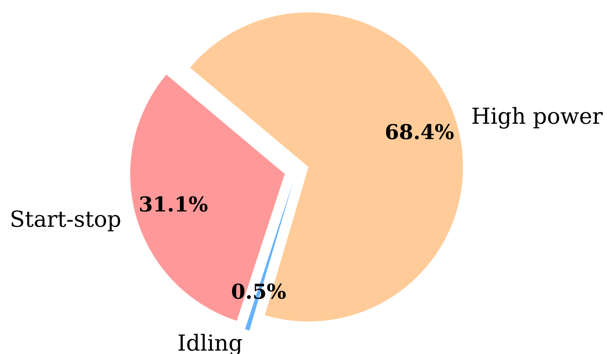
PEMWE Degradation
