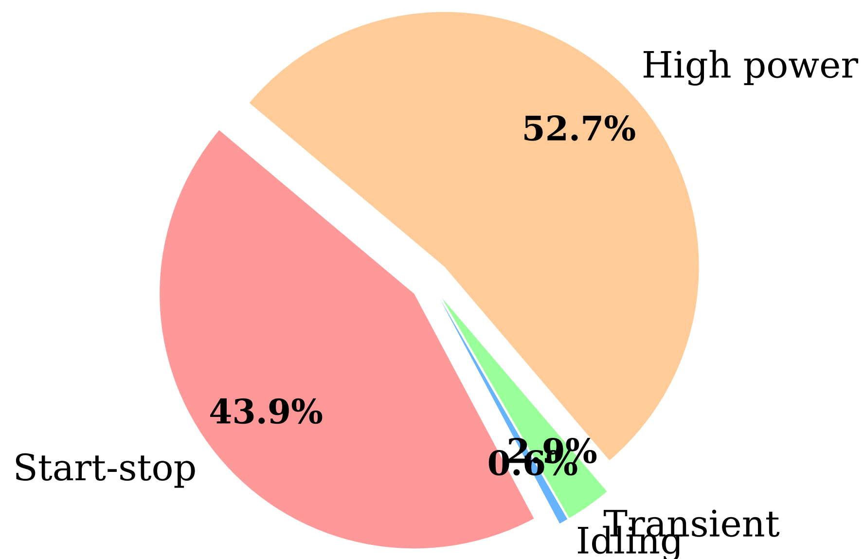
PEMFC Degradation
