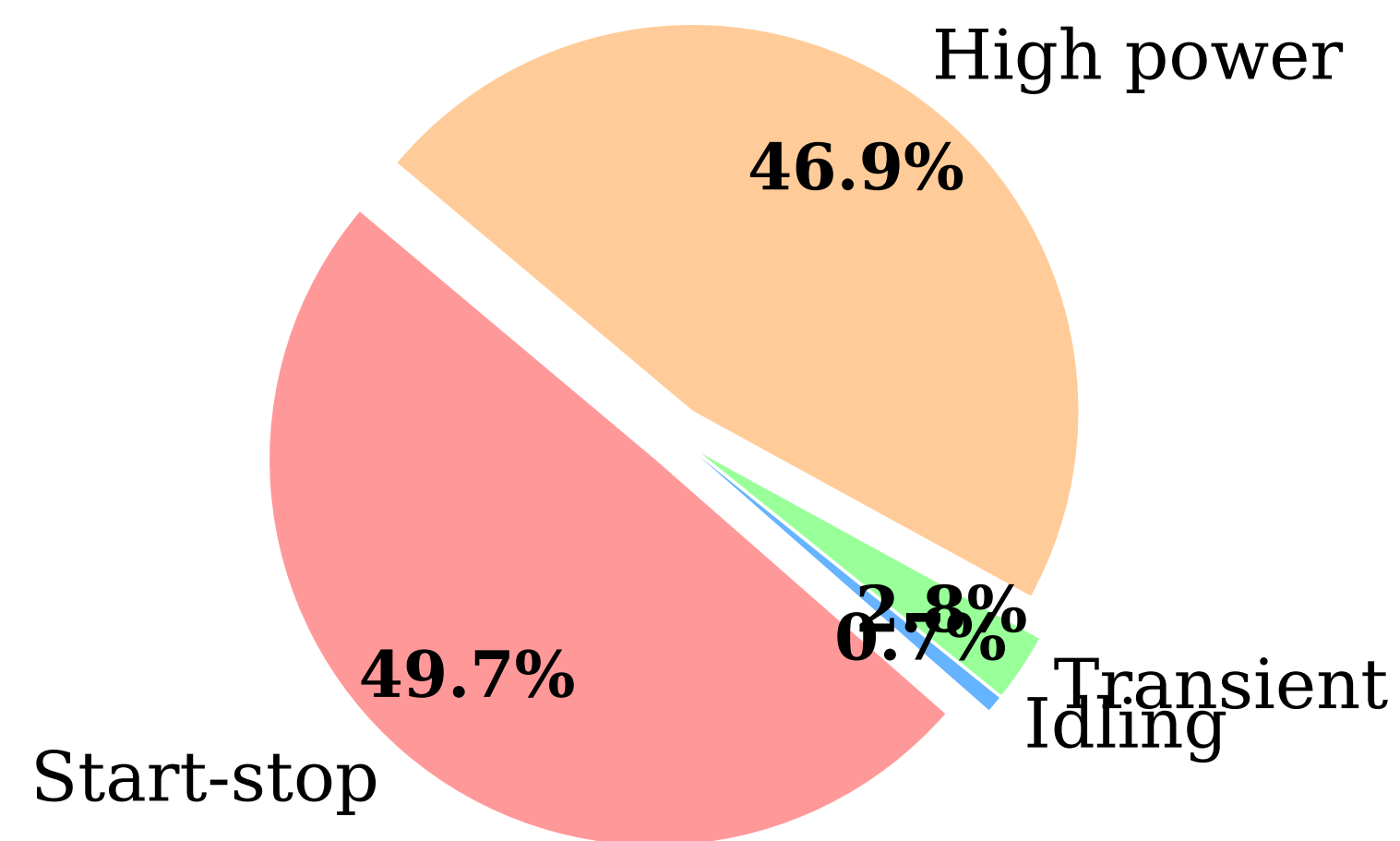
PEMFC Degradation
