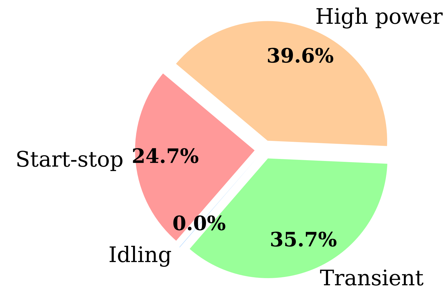
PEMWE Degradation
