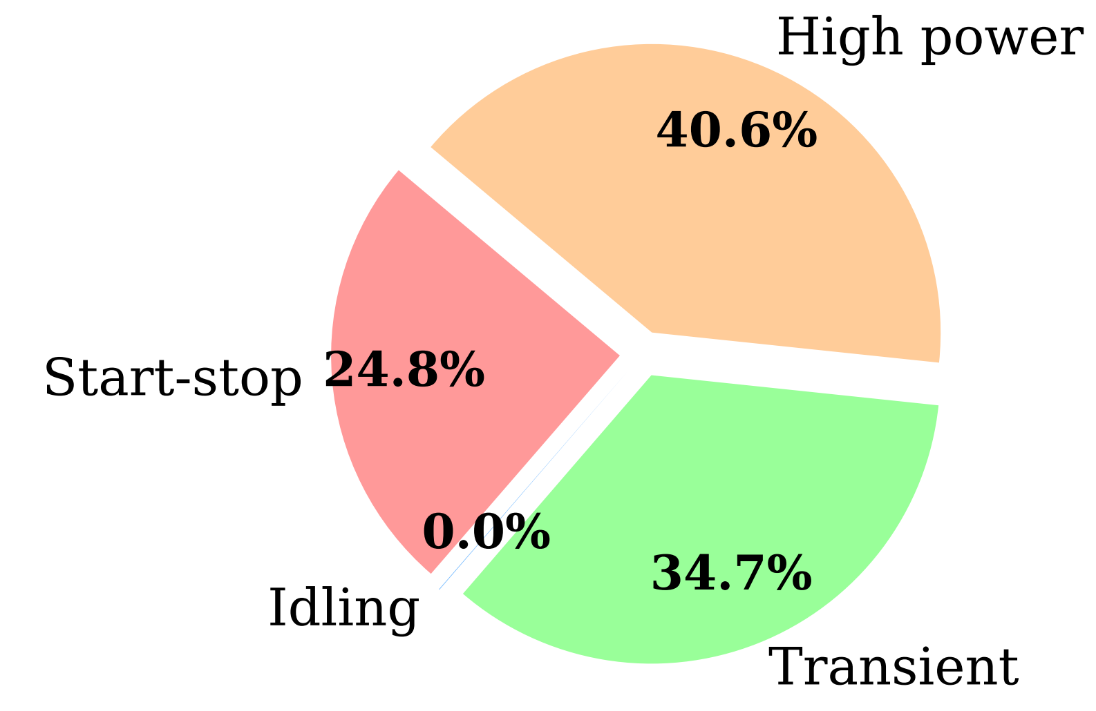
PEMWE Degradation
