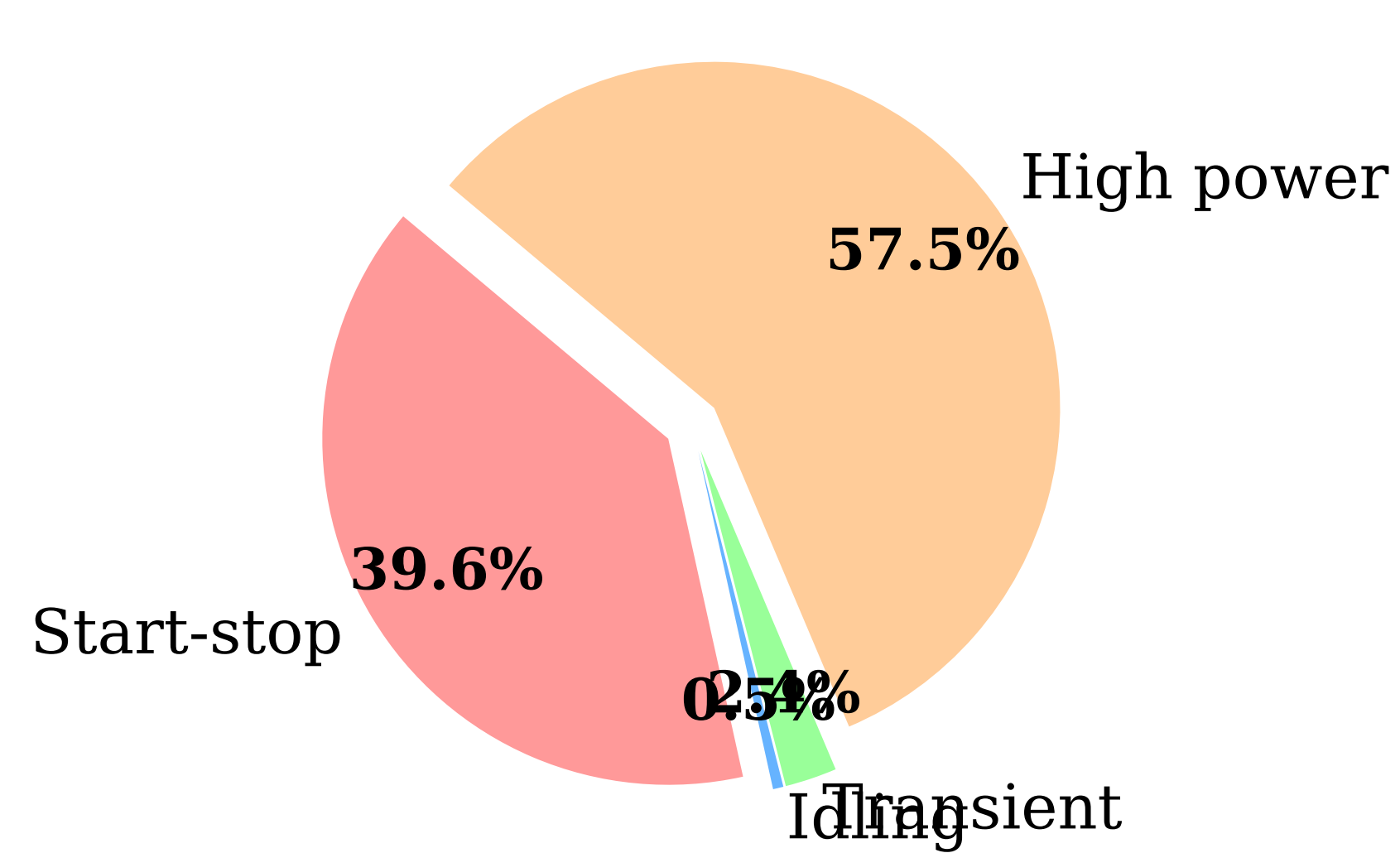
PEMFC Degradation
