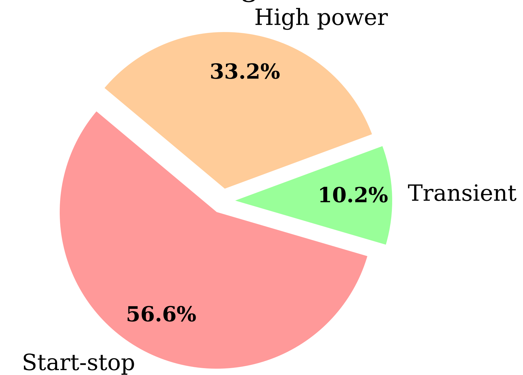
PEMWE Degradation
