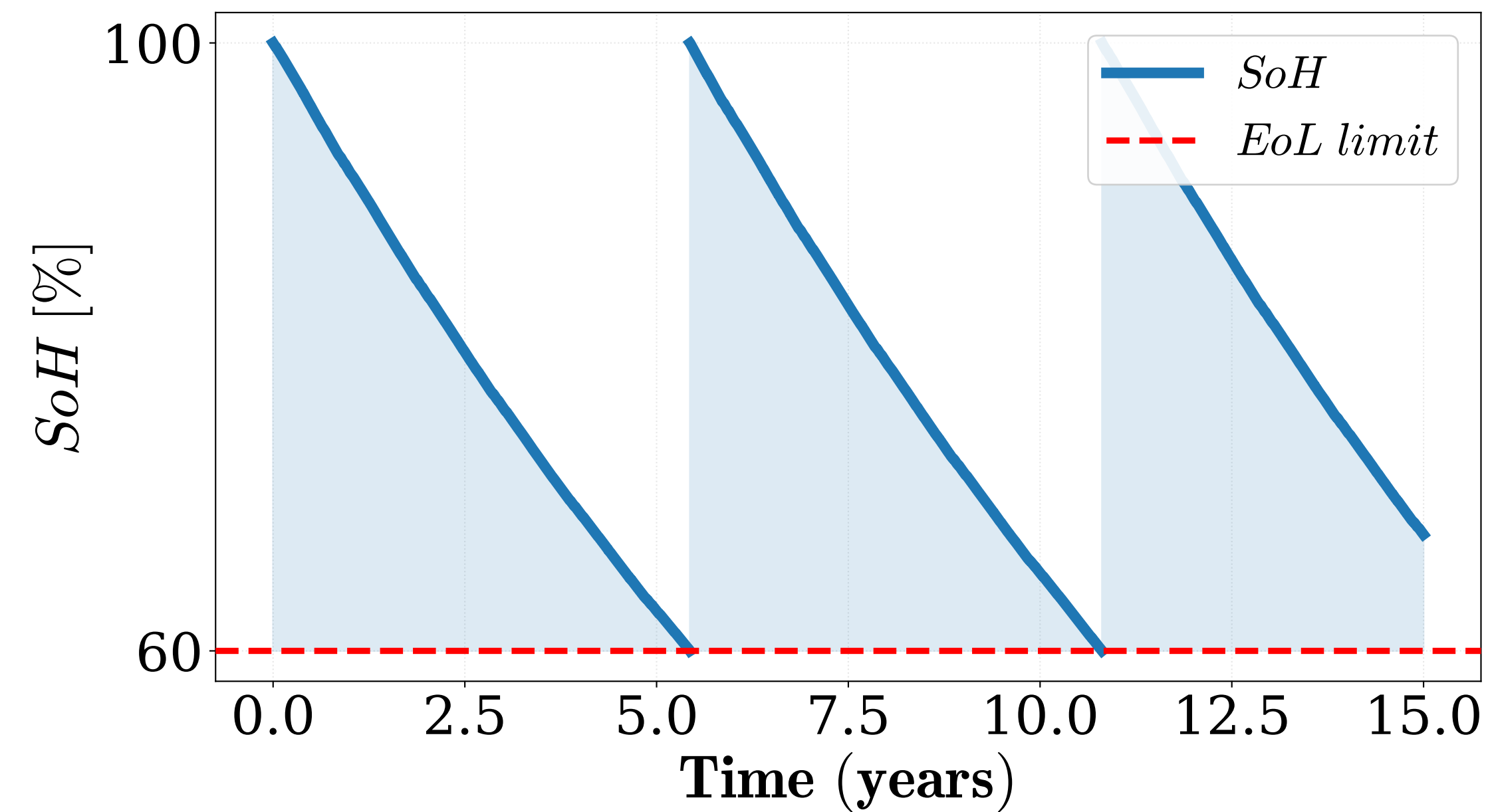
PEMFC Degradation
