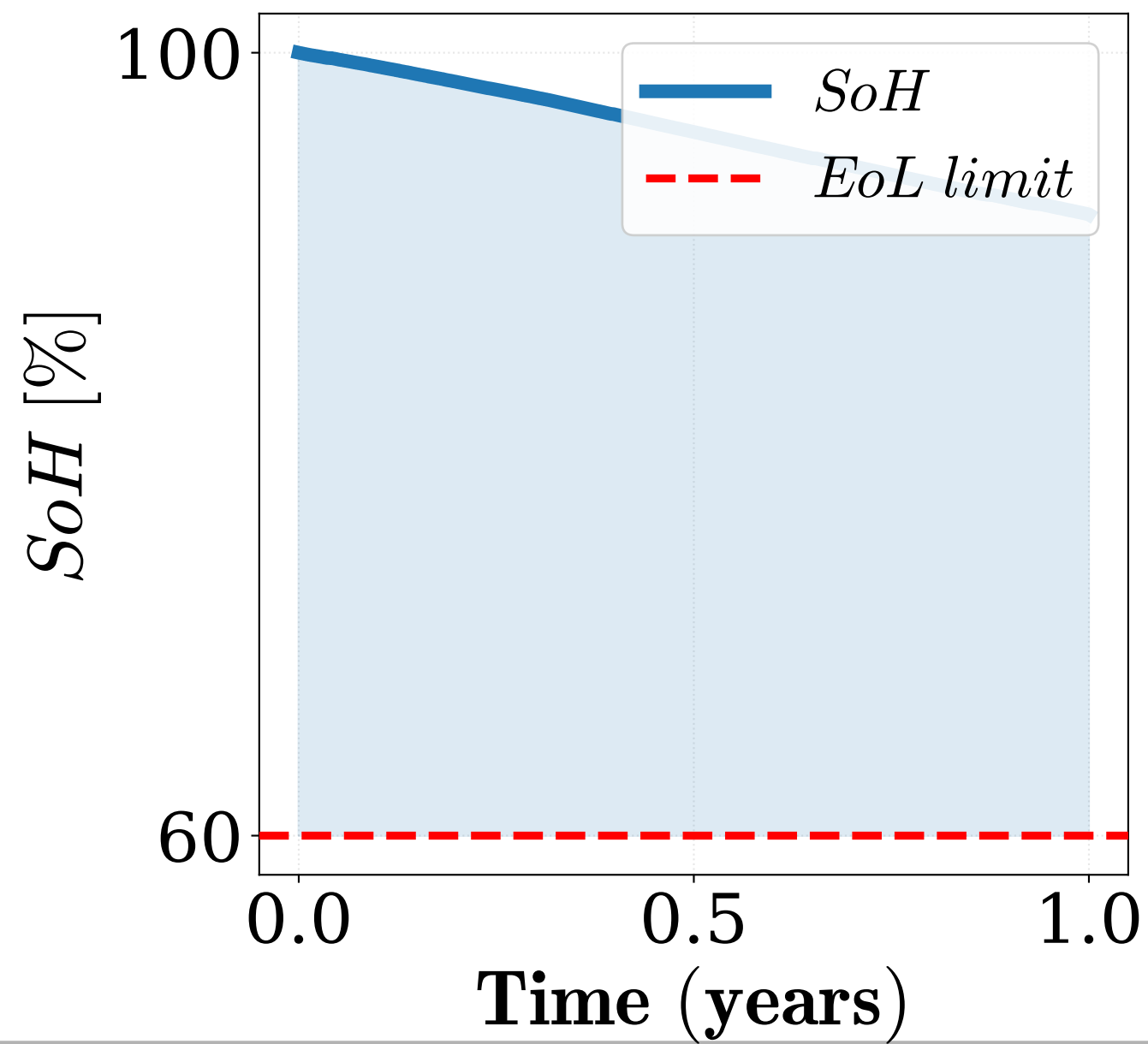
PEMFC Degradation
