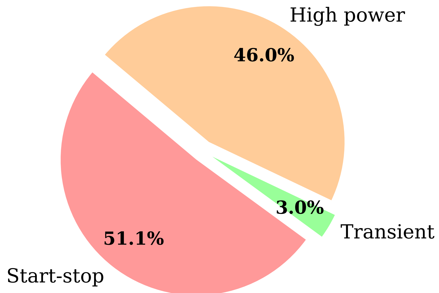
PEMFC Degradation
