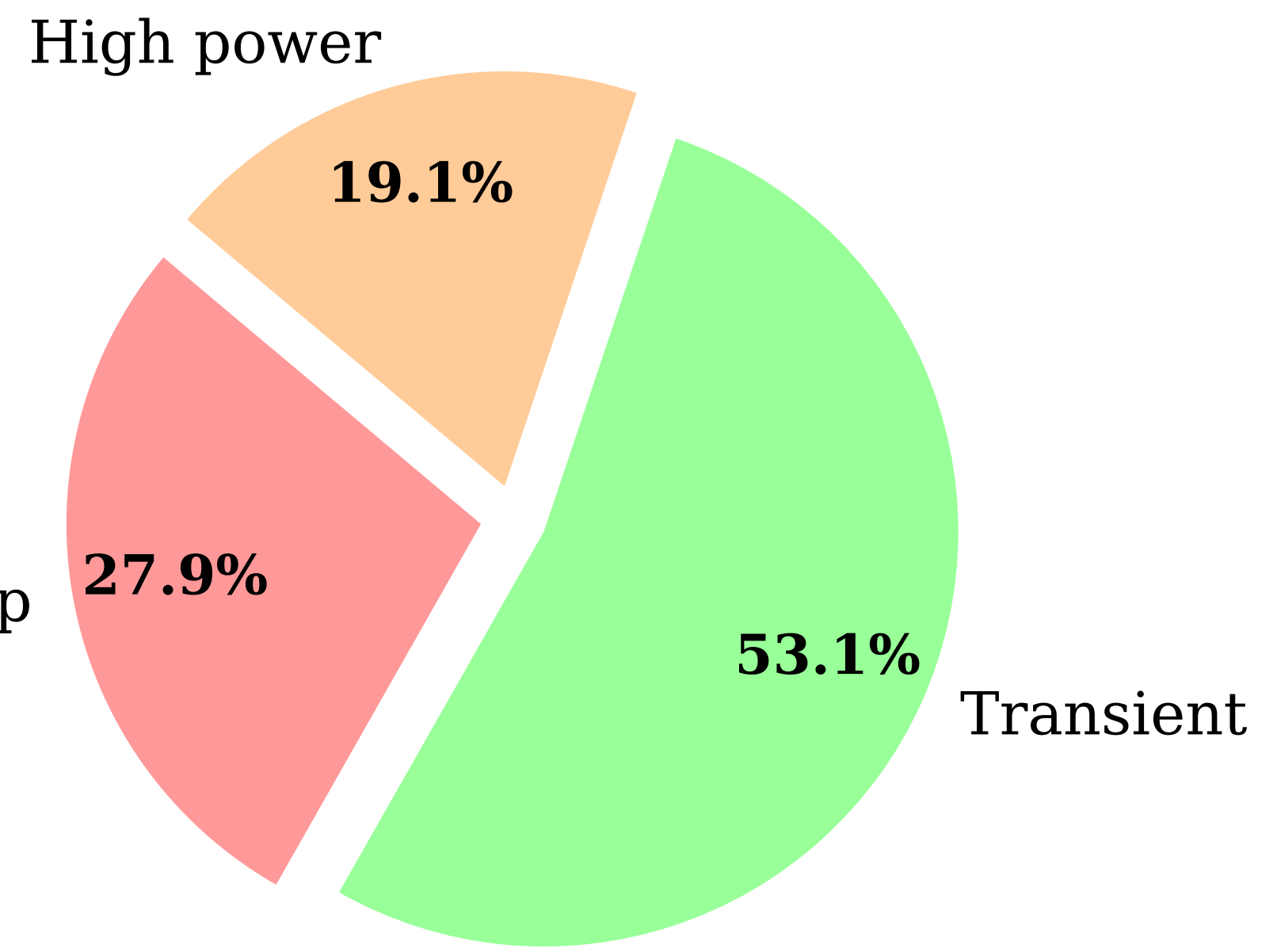
PEMWE Degradation
