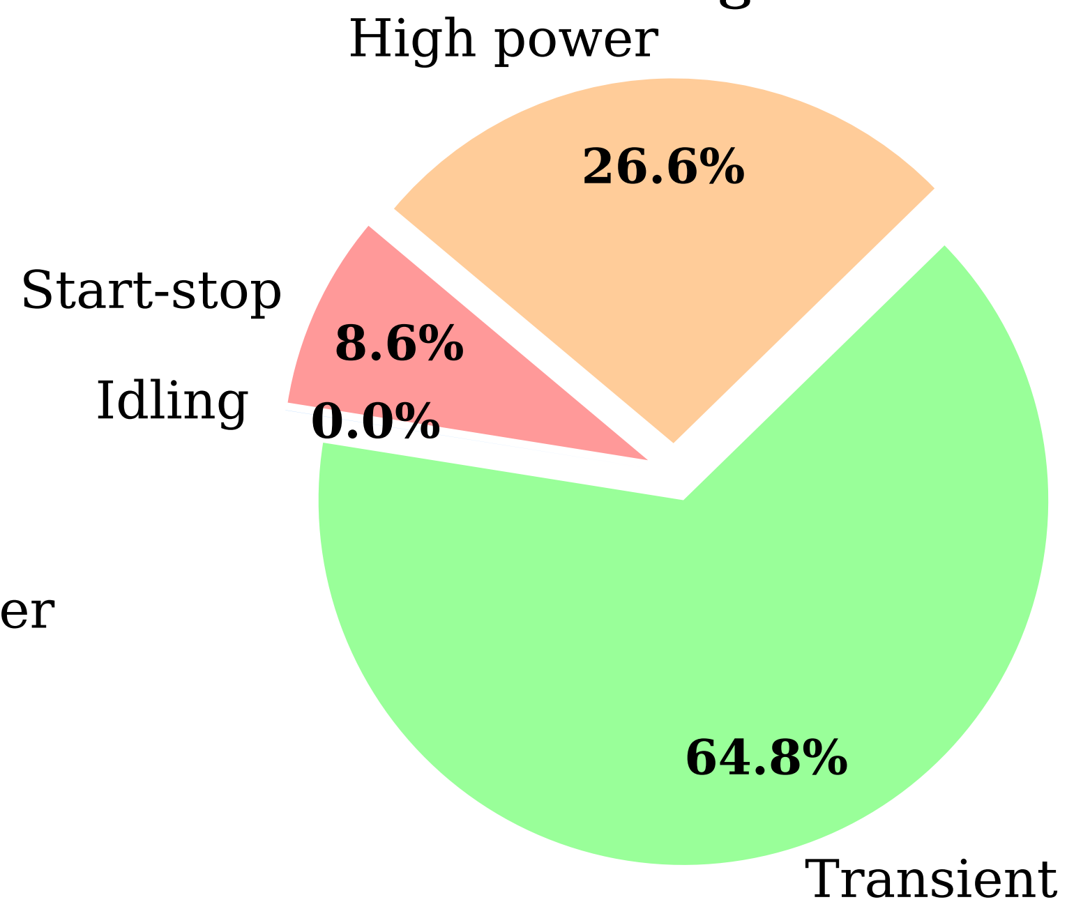
PEMWE Degradation
