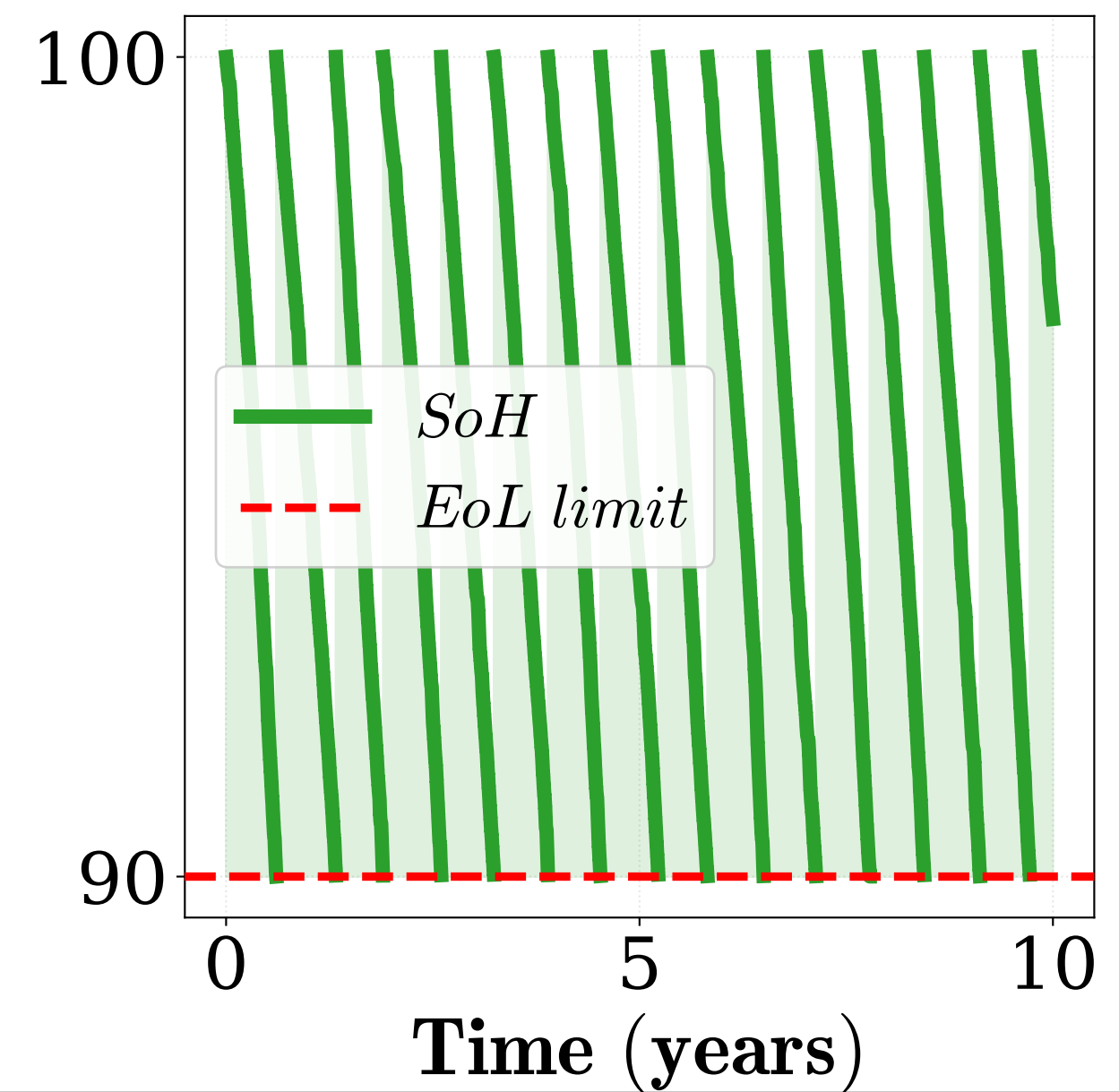
PEMWE Degradation
