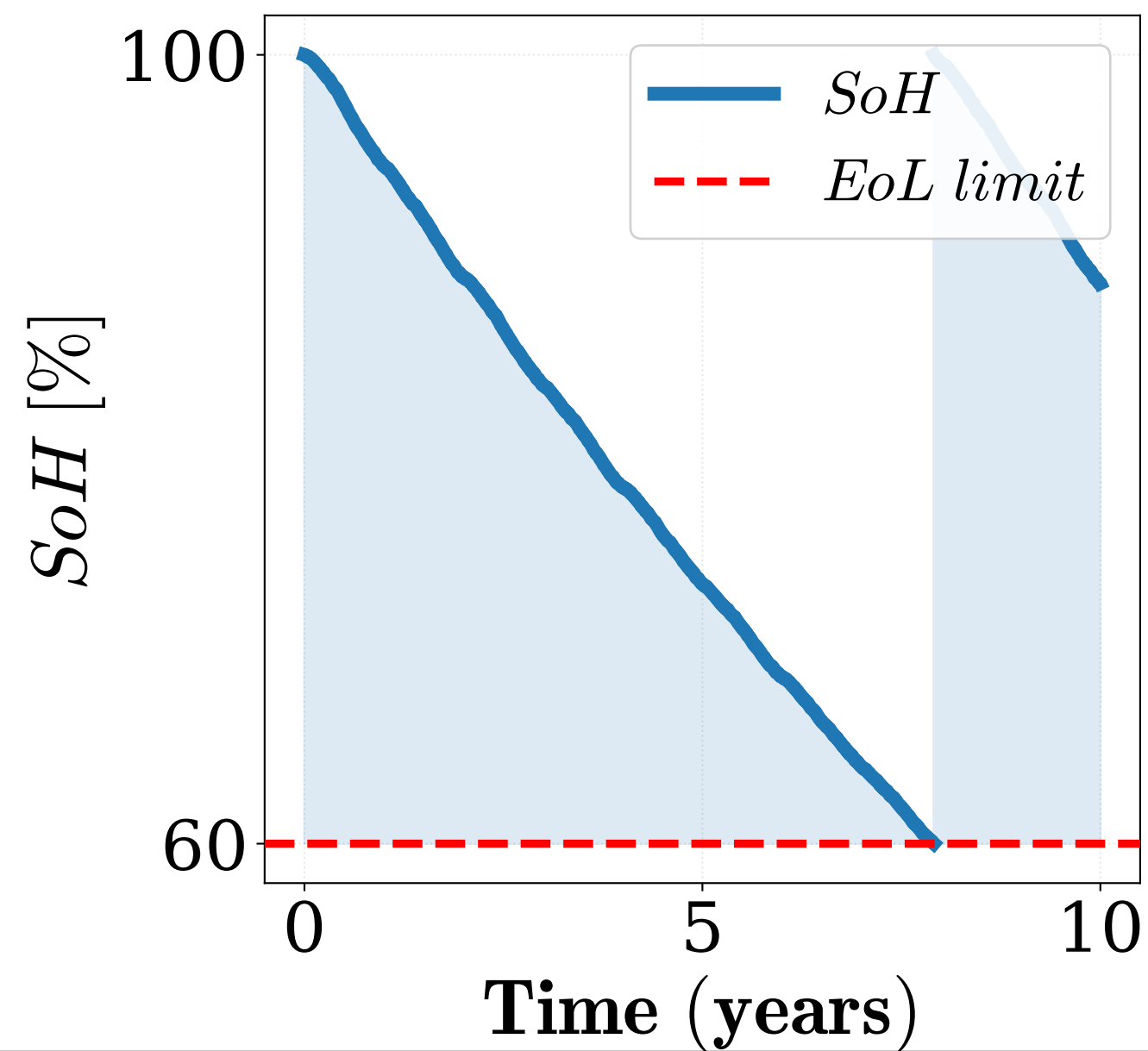
PEMFC Degradation
