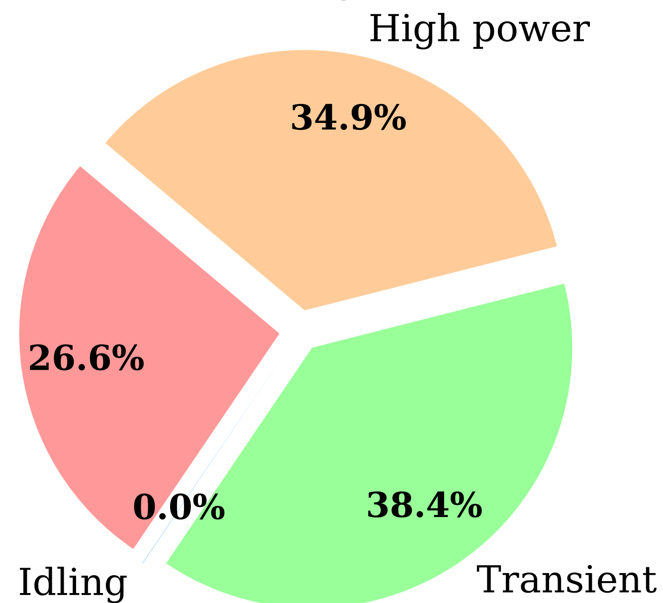
PEMWE Degradation
