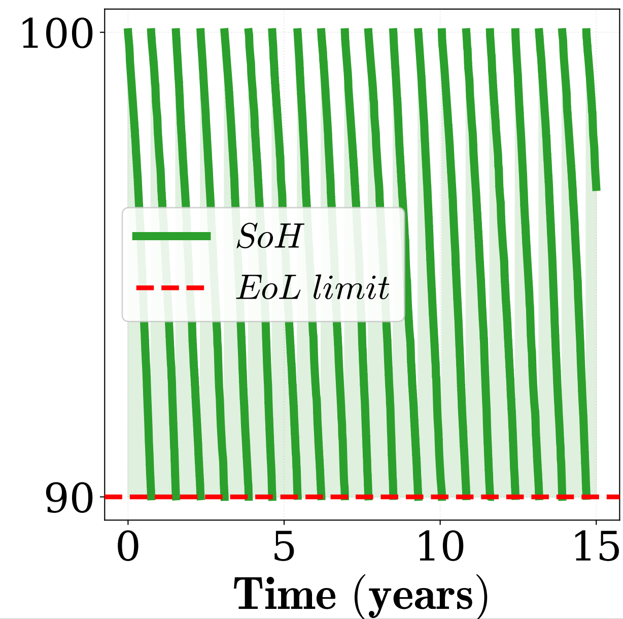
PEMWE Degradation
