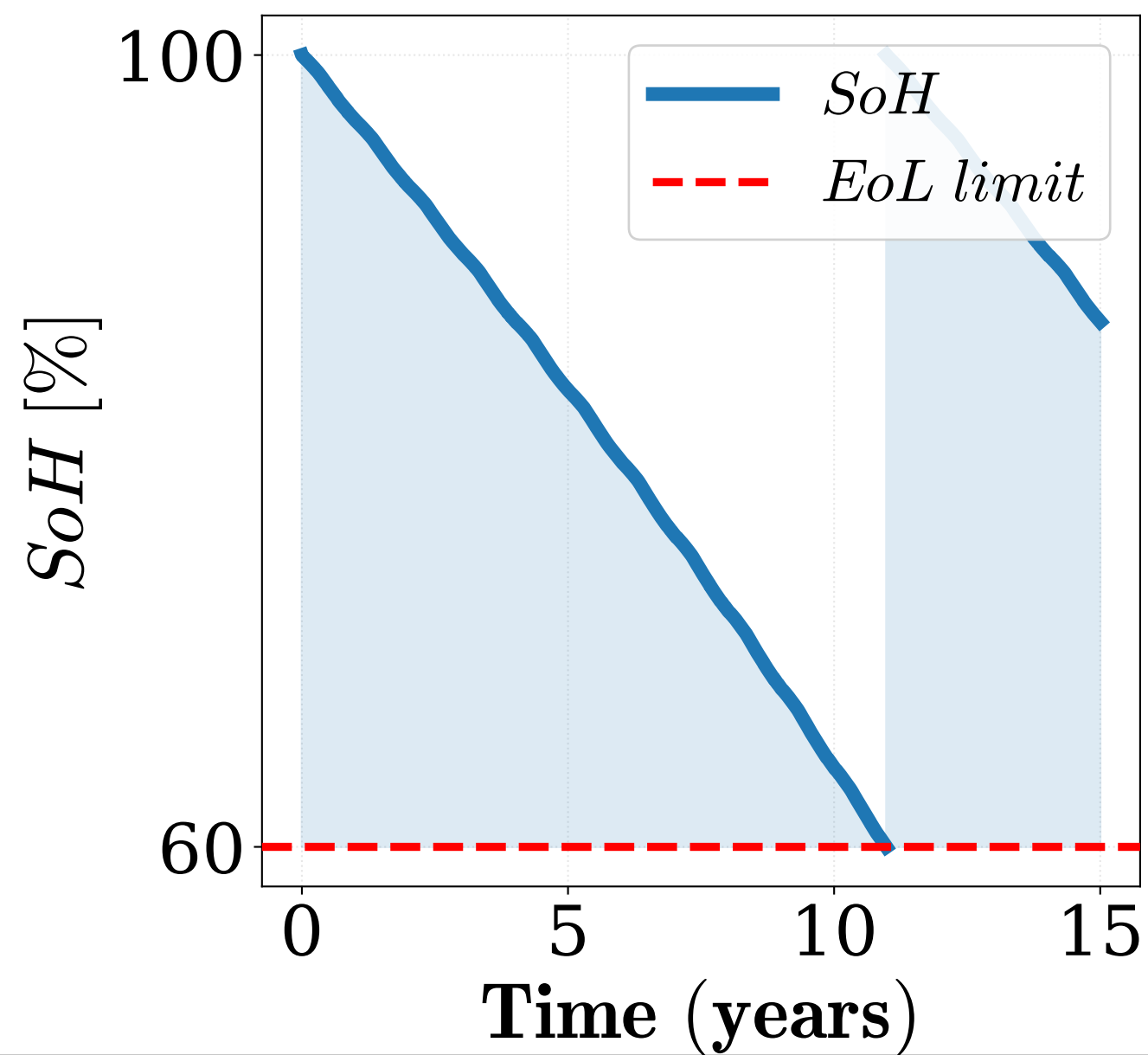
PEMFC Degradation
