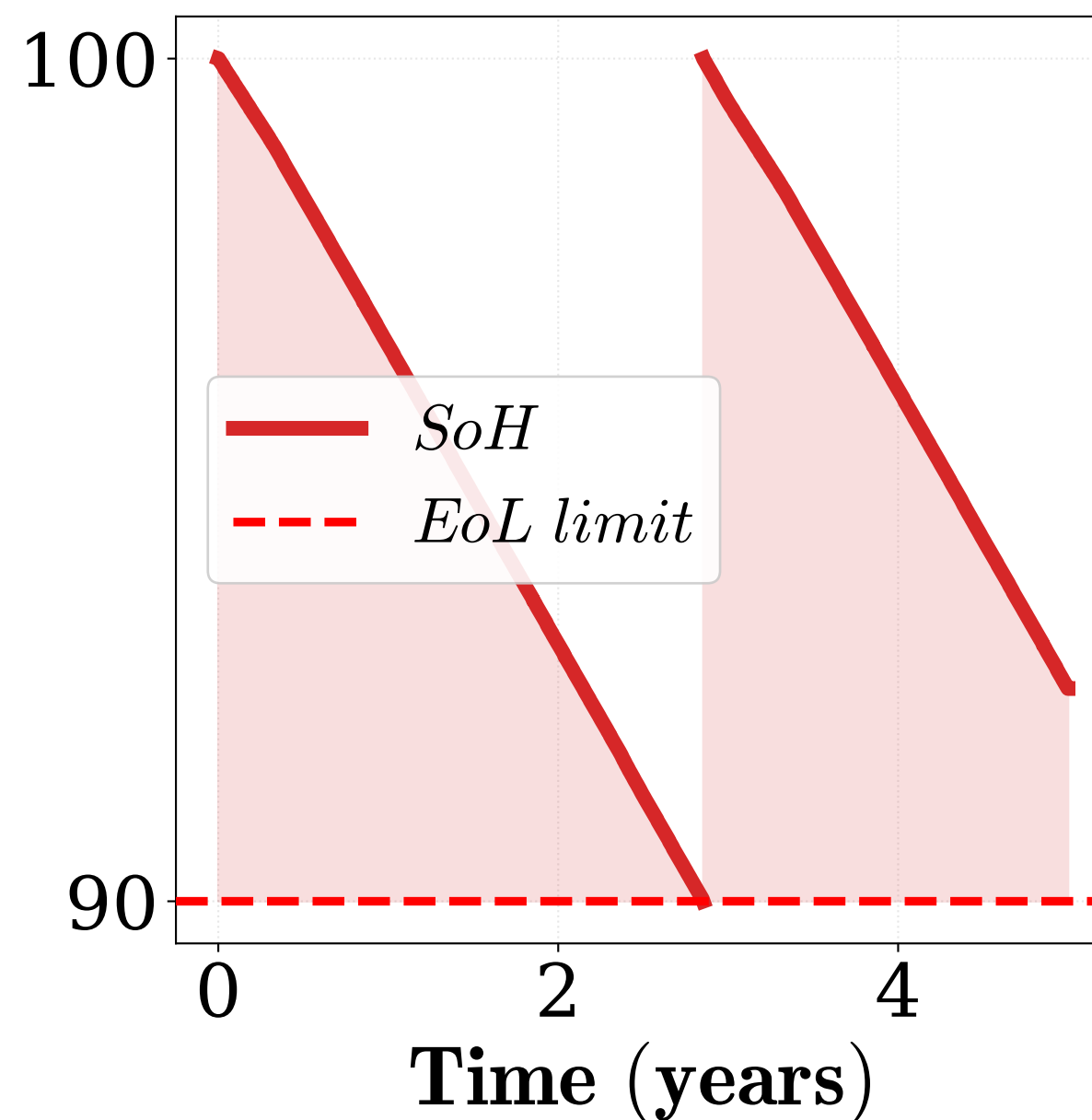
PEMFC
