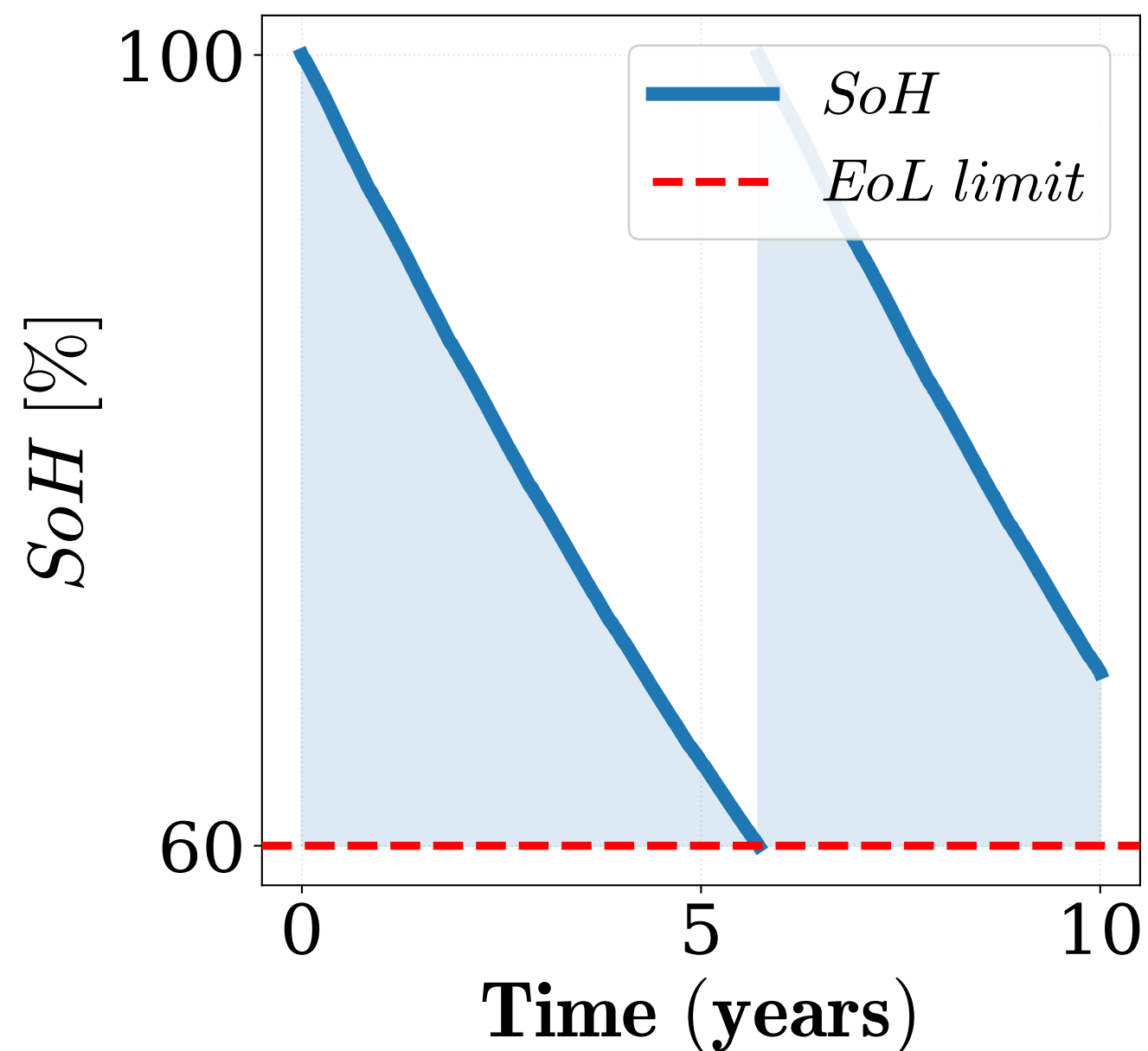
PEMFC Degradation
