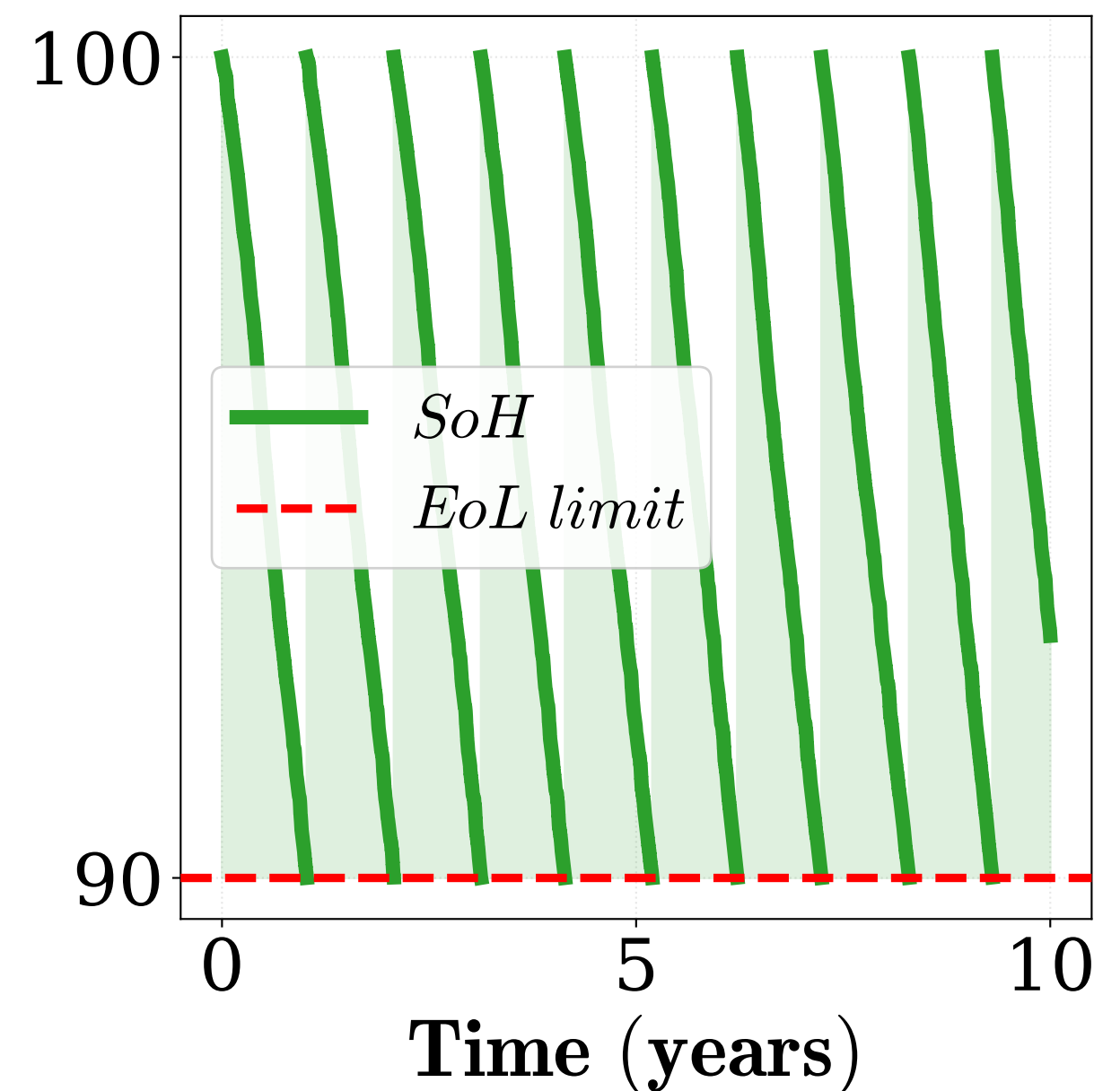
PEMWE Degradation
