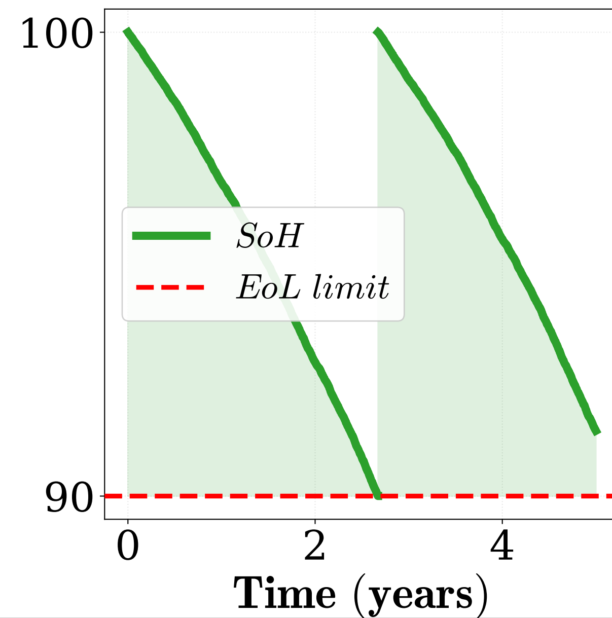
PEMWE Degradation
