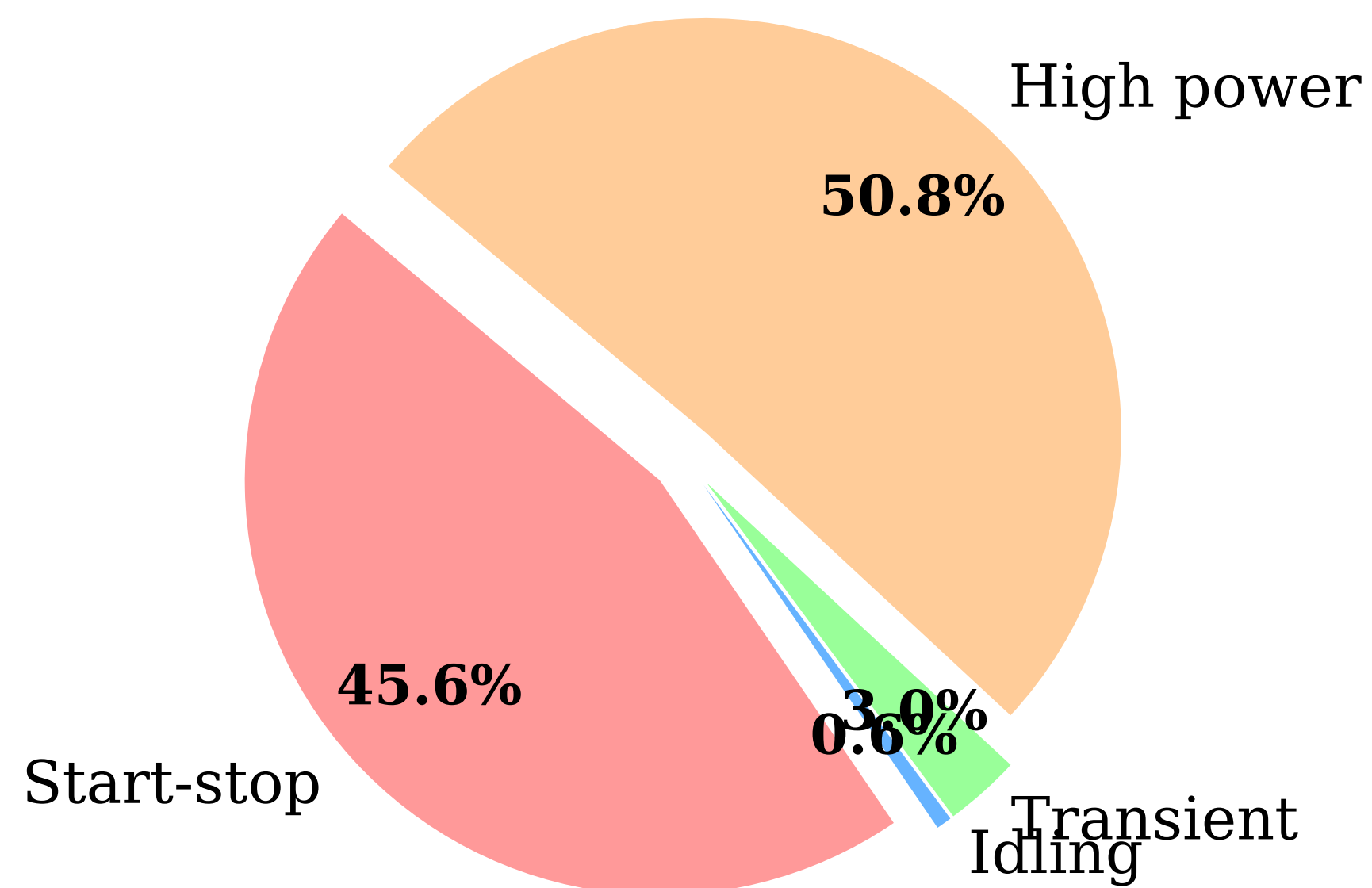
PEMFC Degradation
