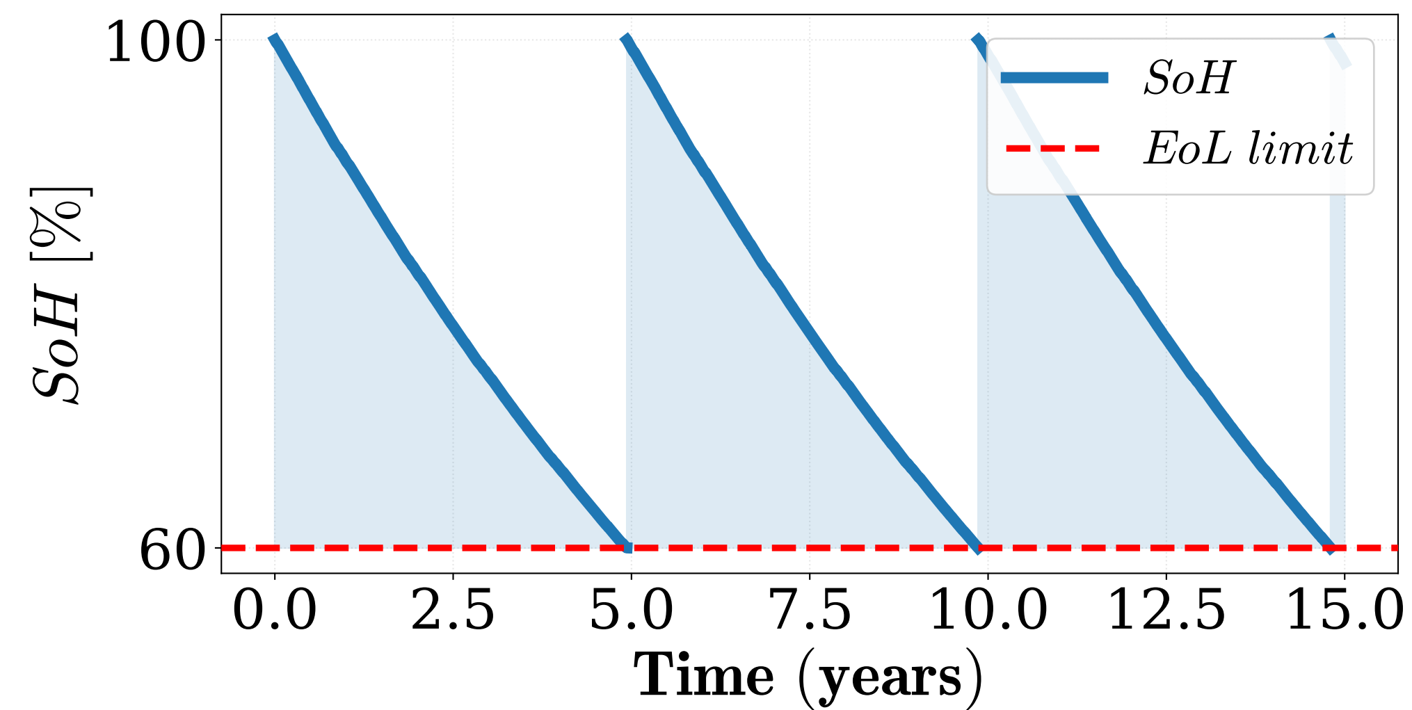
PEMFC Degradation
