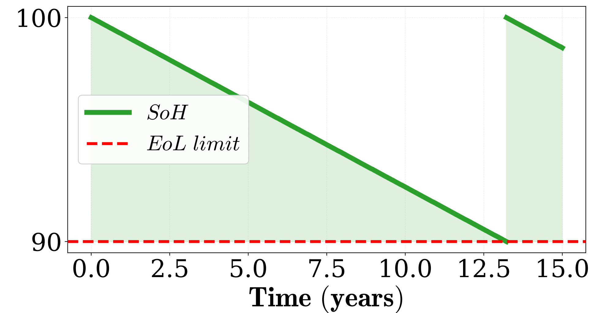
PEMWE Degradation
