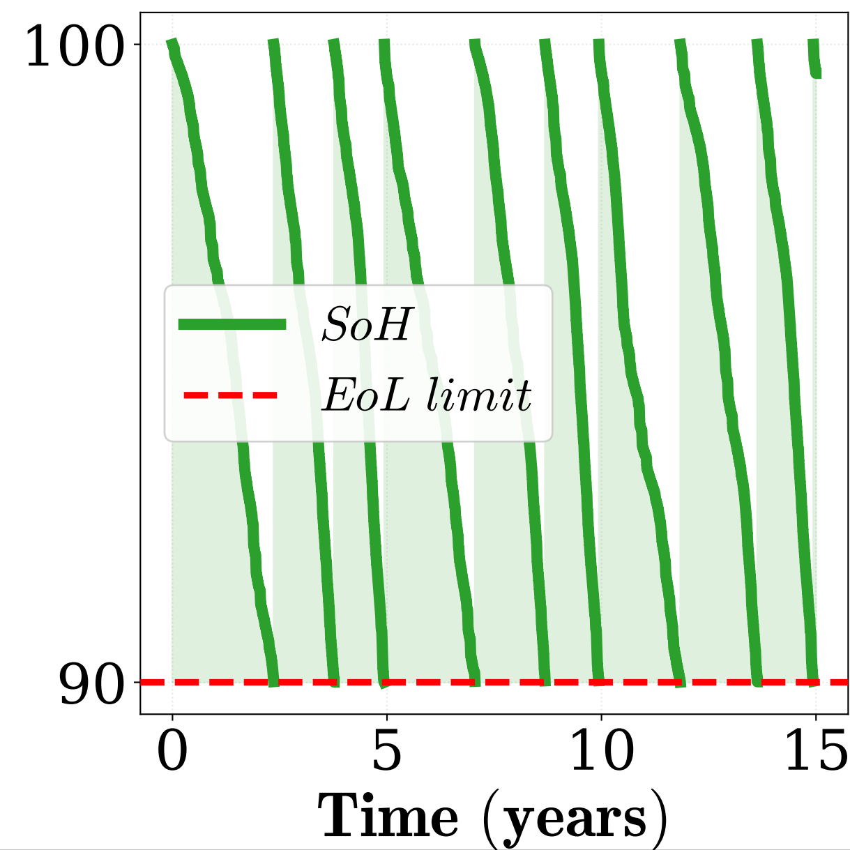
PEMWE Degradation
