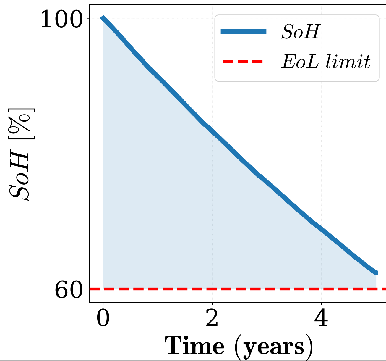
PEMFC Degradation
