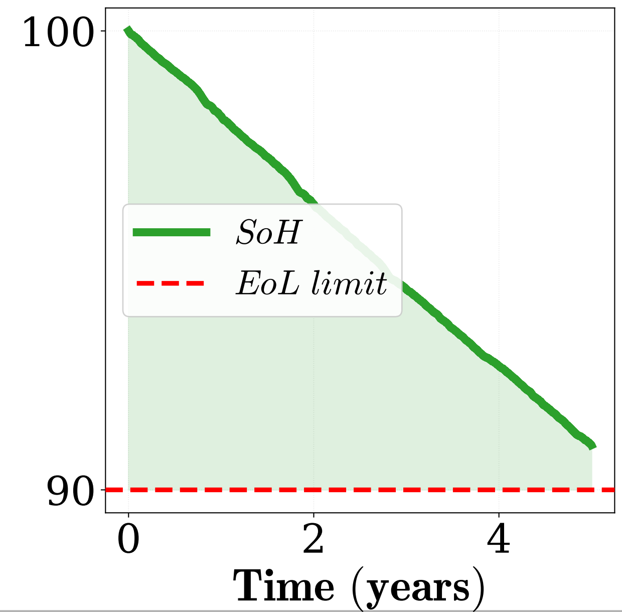
PEMWE Degradation
