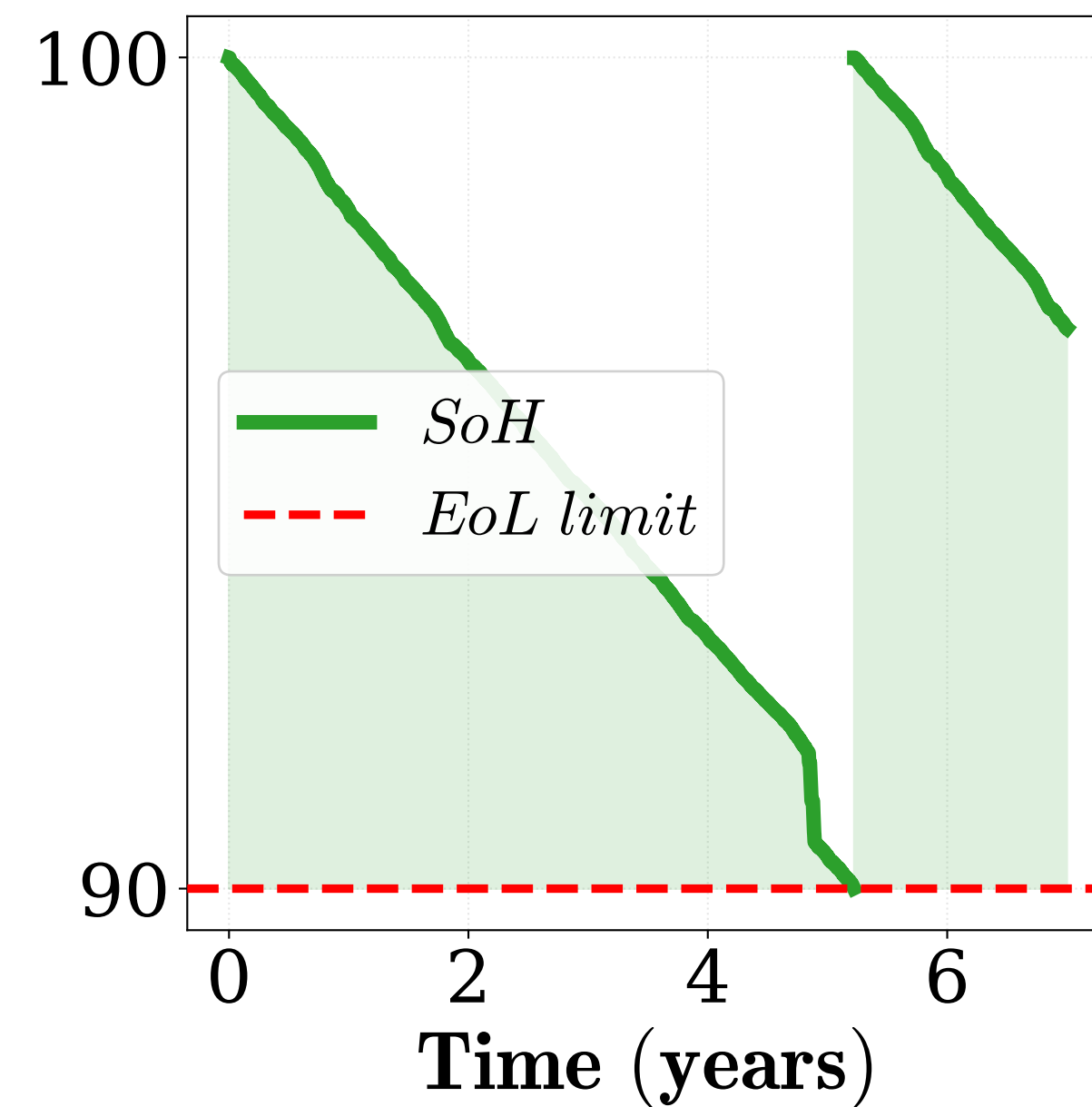
PEMWE Degradation
