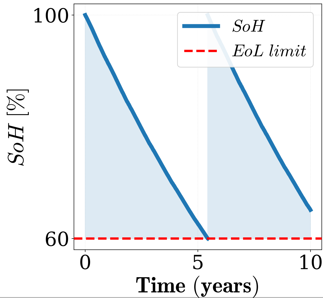
PEMFC Degradation
