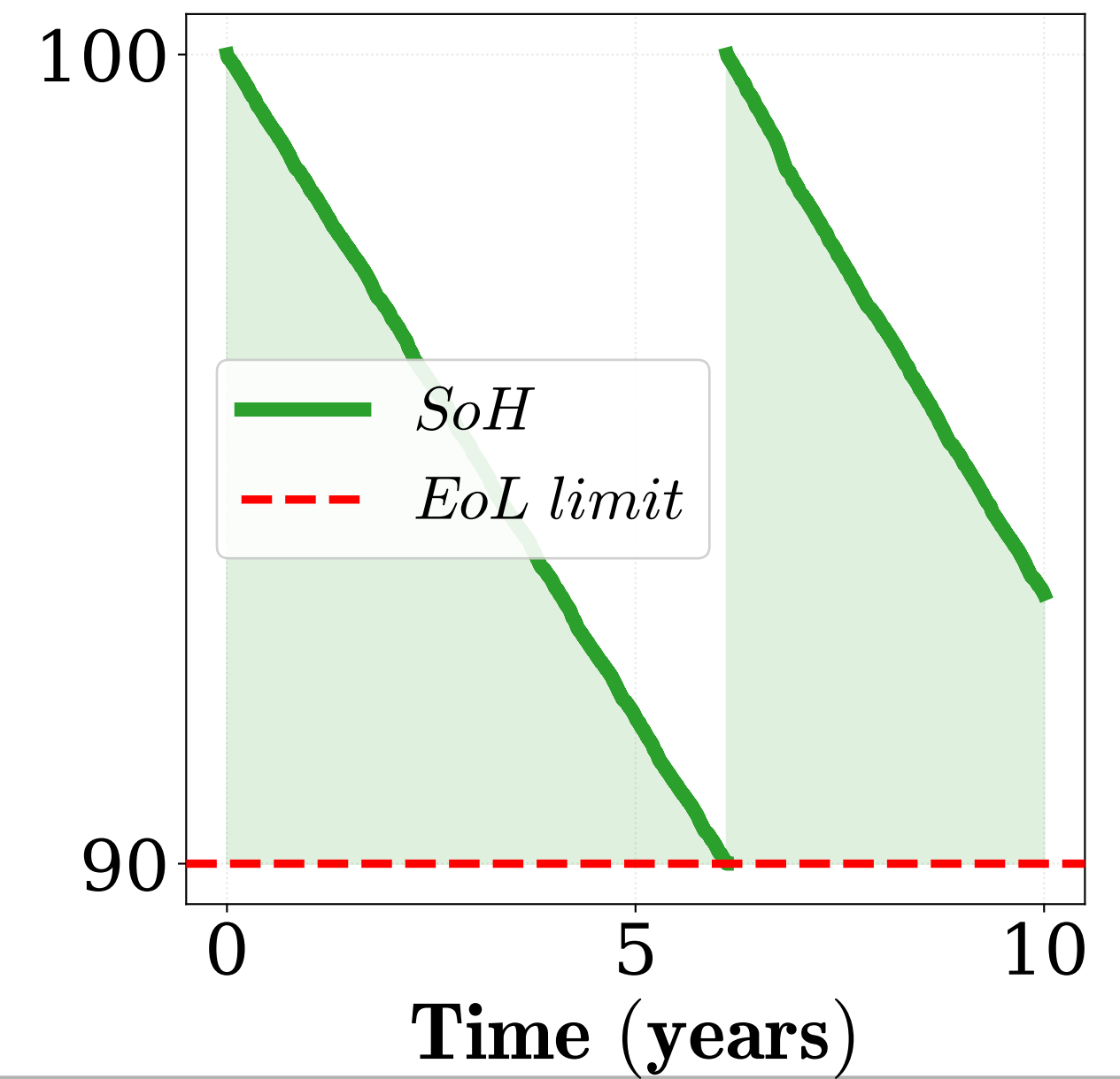
PEMWE Degradation
