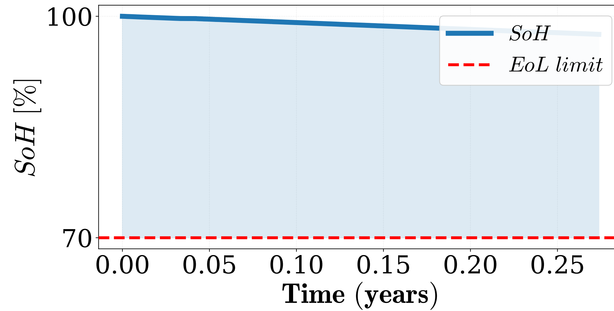
PEMFC Degradation
