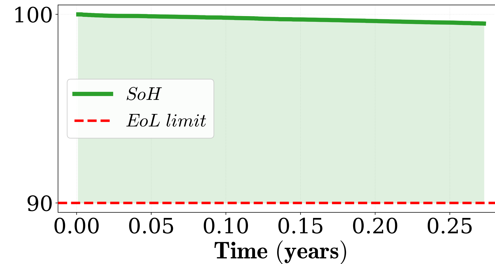
PEMWE Degradation
