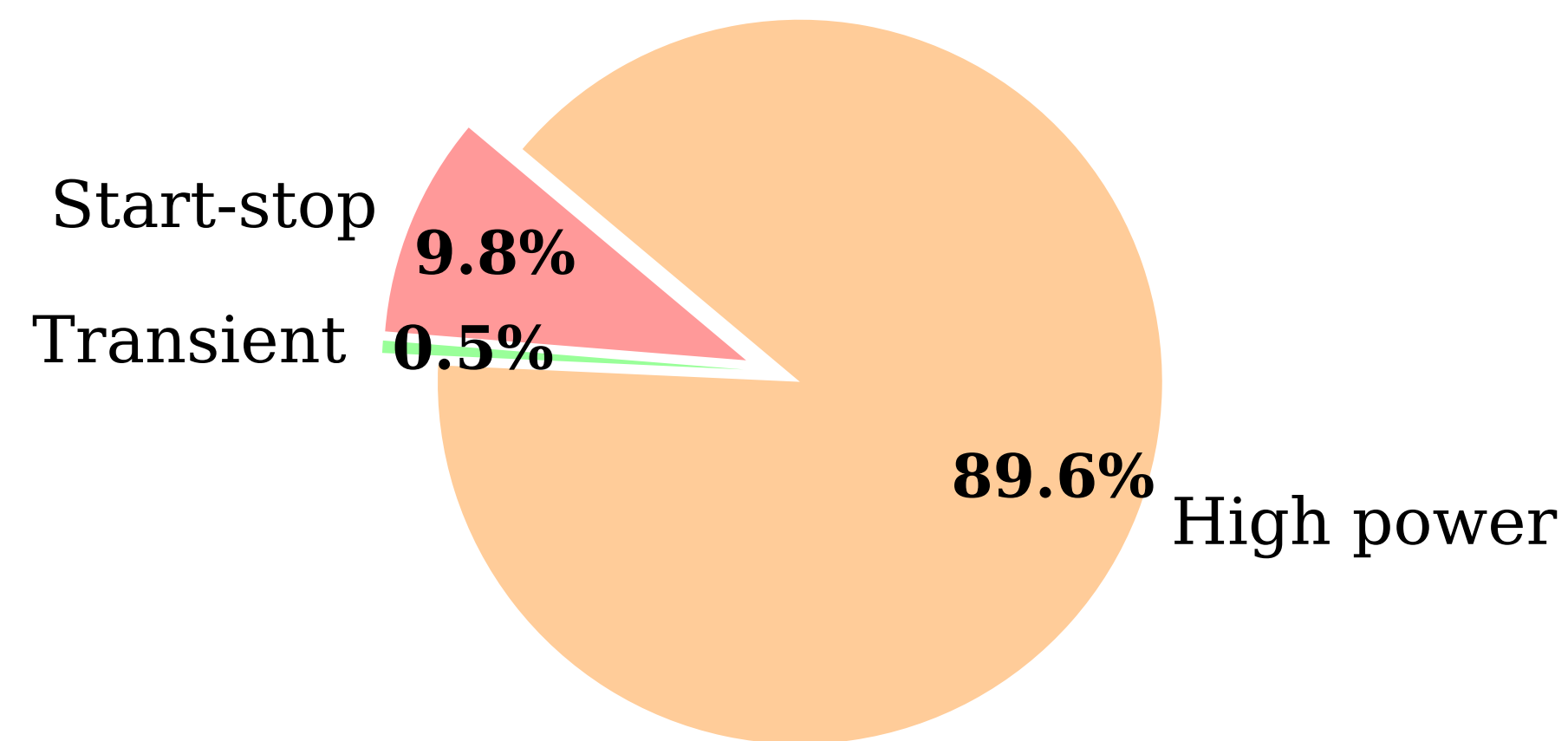
PEMFC Degradation
