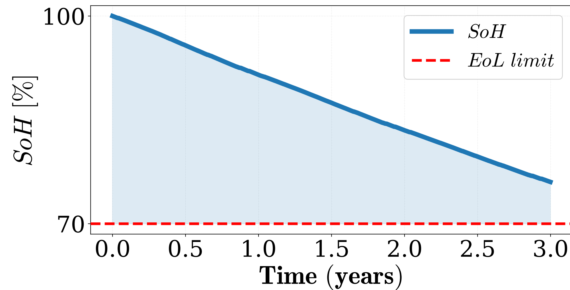
PEMFC Degradation
