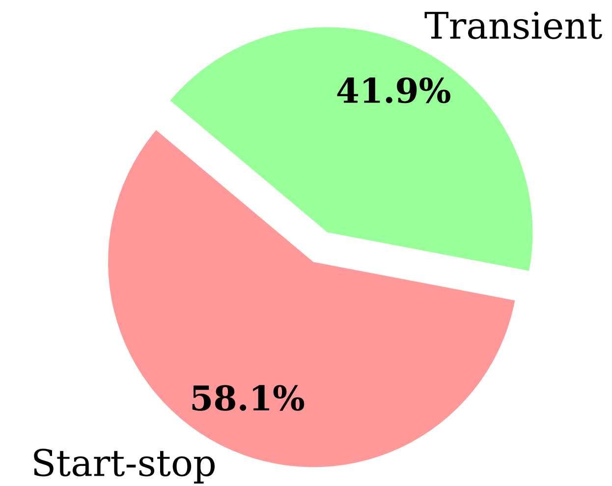
PEMWE Degradation
