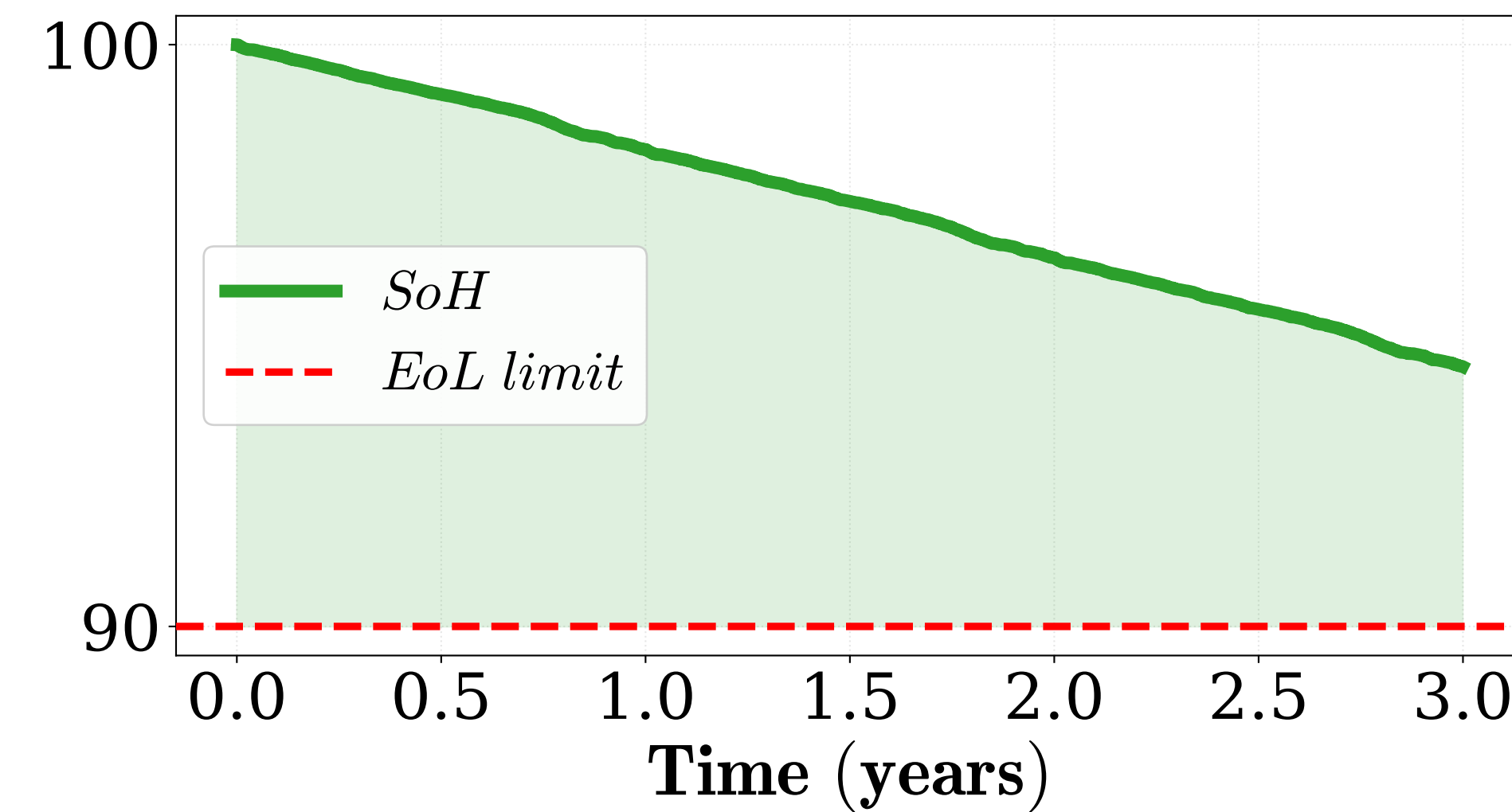
PEMWE Degradation
