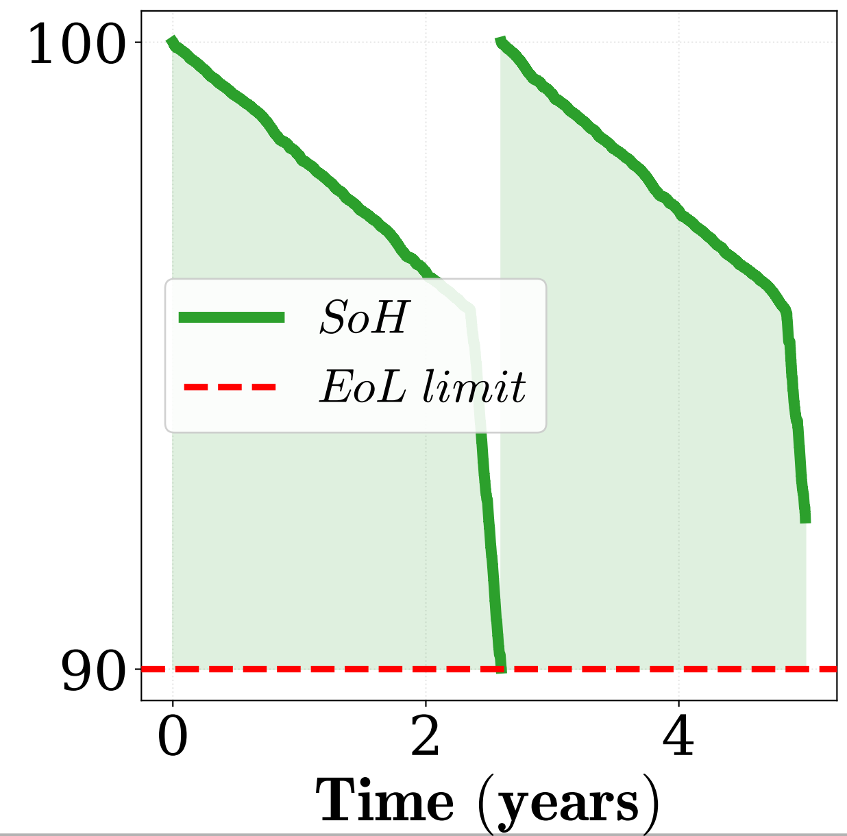
PEMWE Degradation
