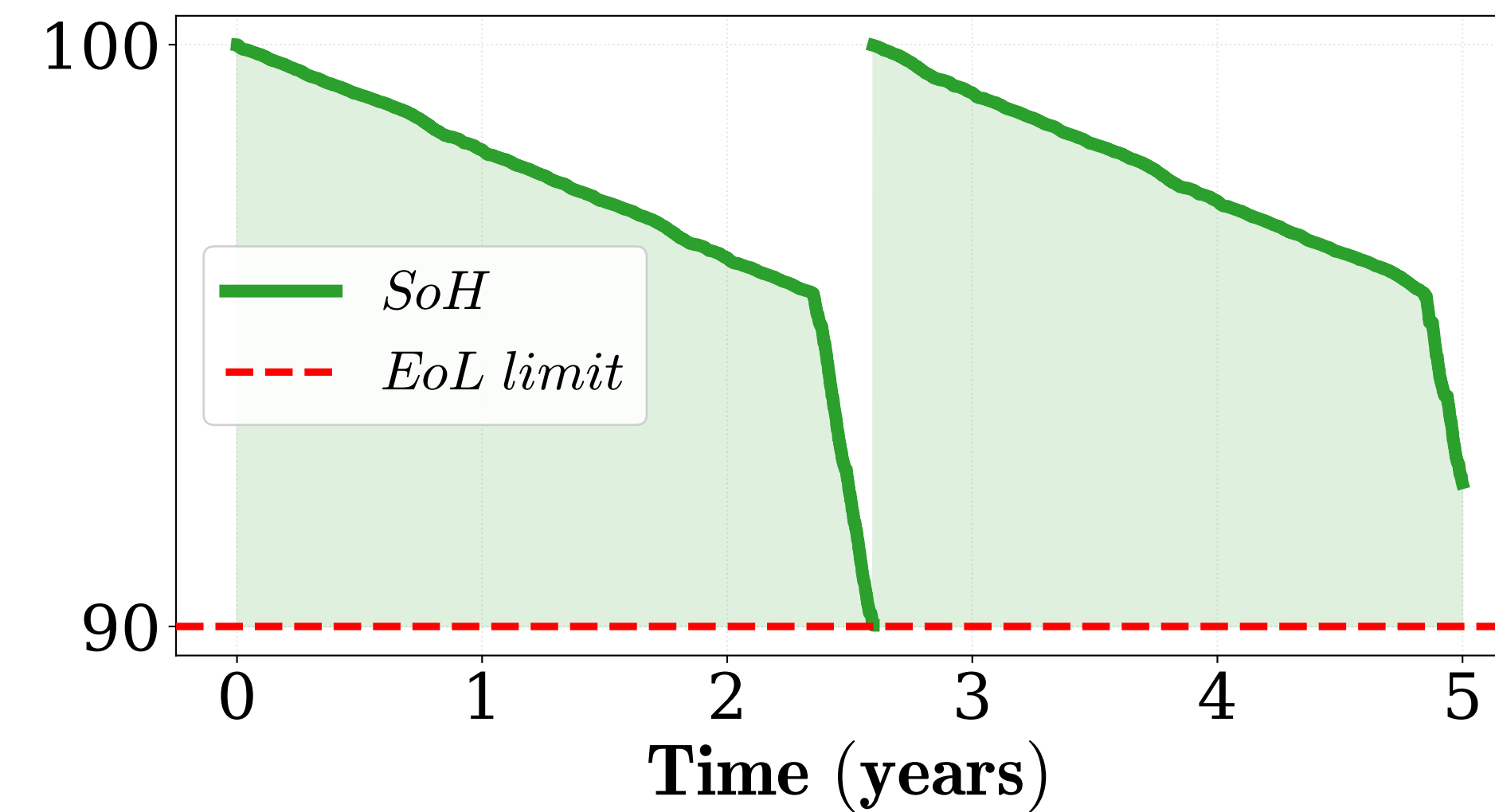
PEMWE Degradation
