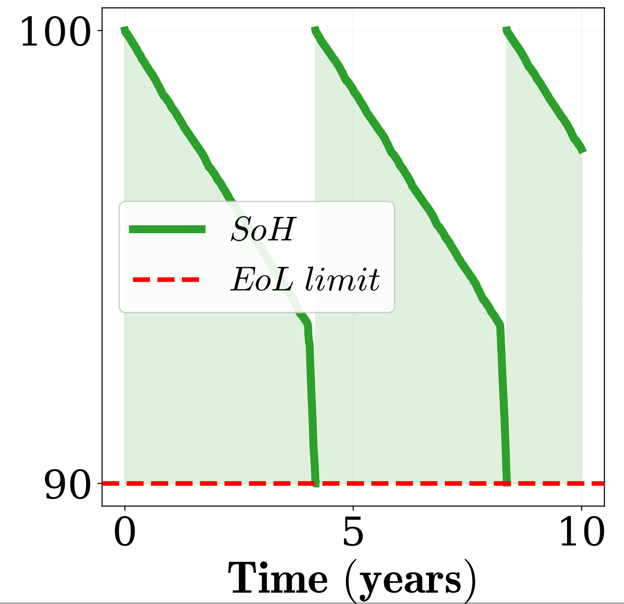
PEMWE Degradation
