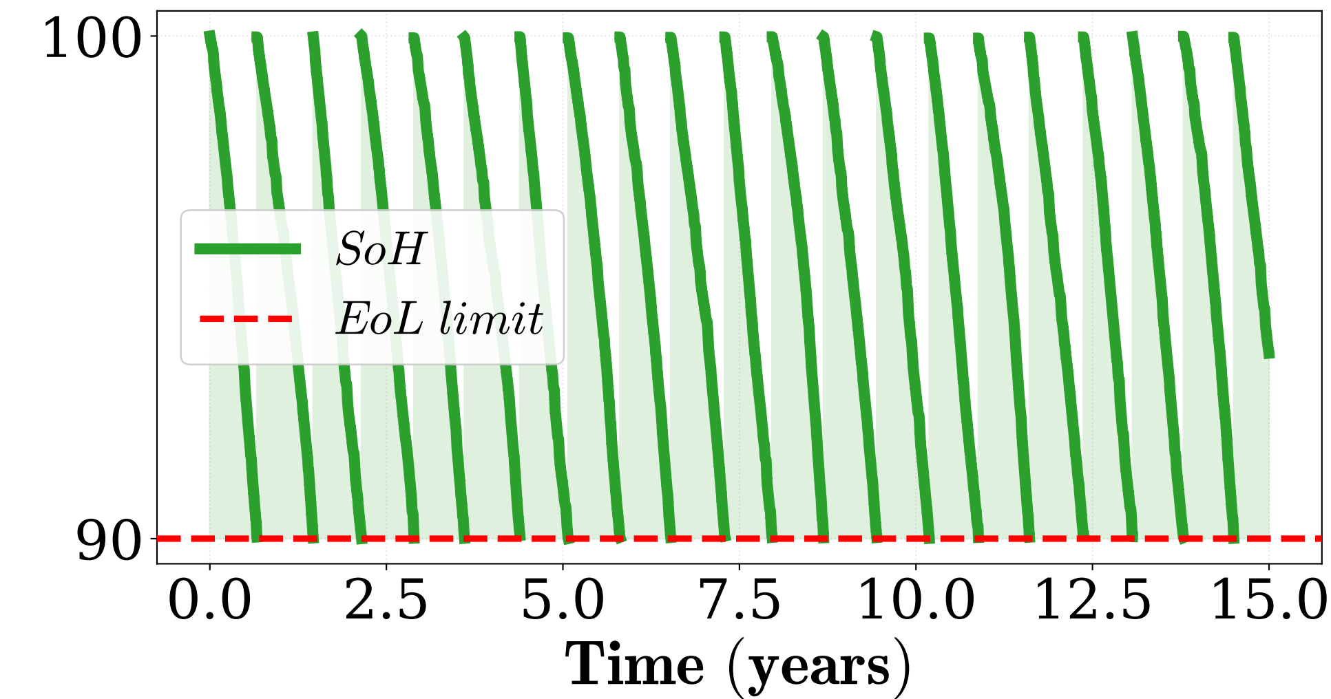
PEMWE Degradation
