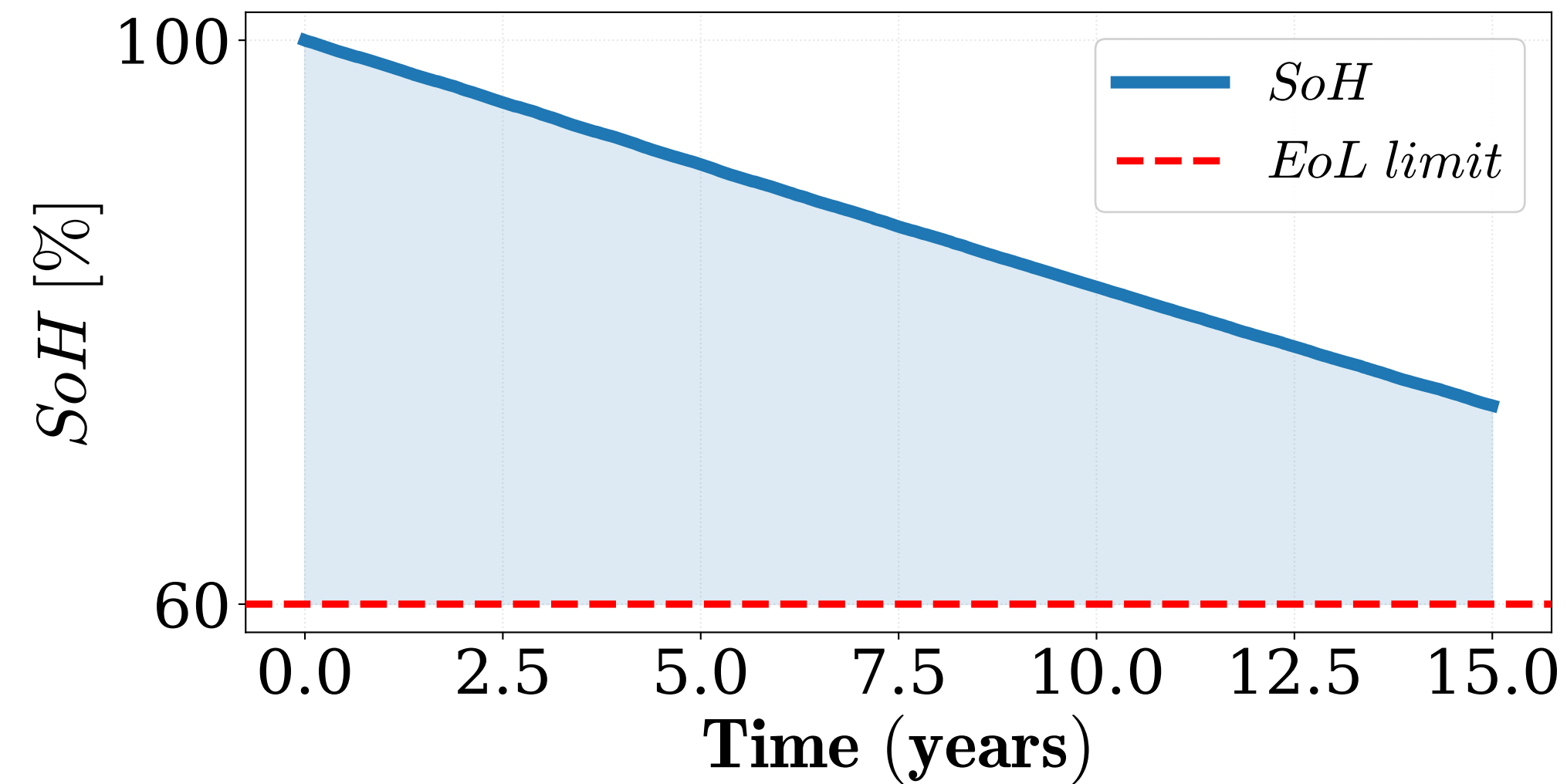
PEMFC Degradation
