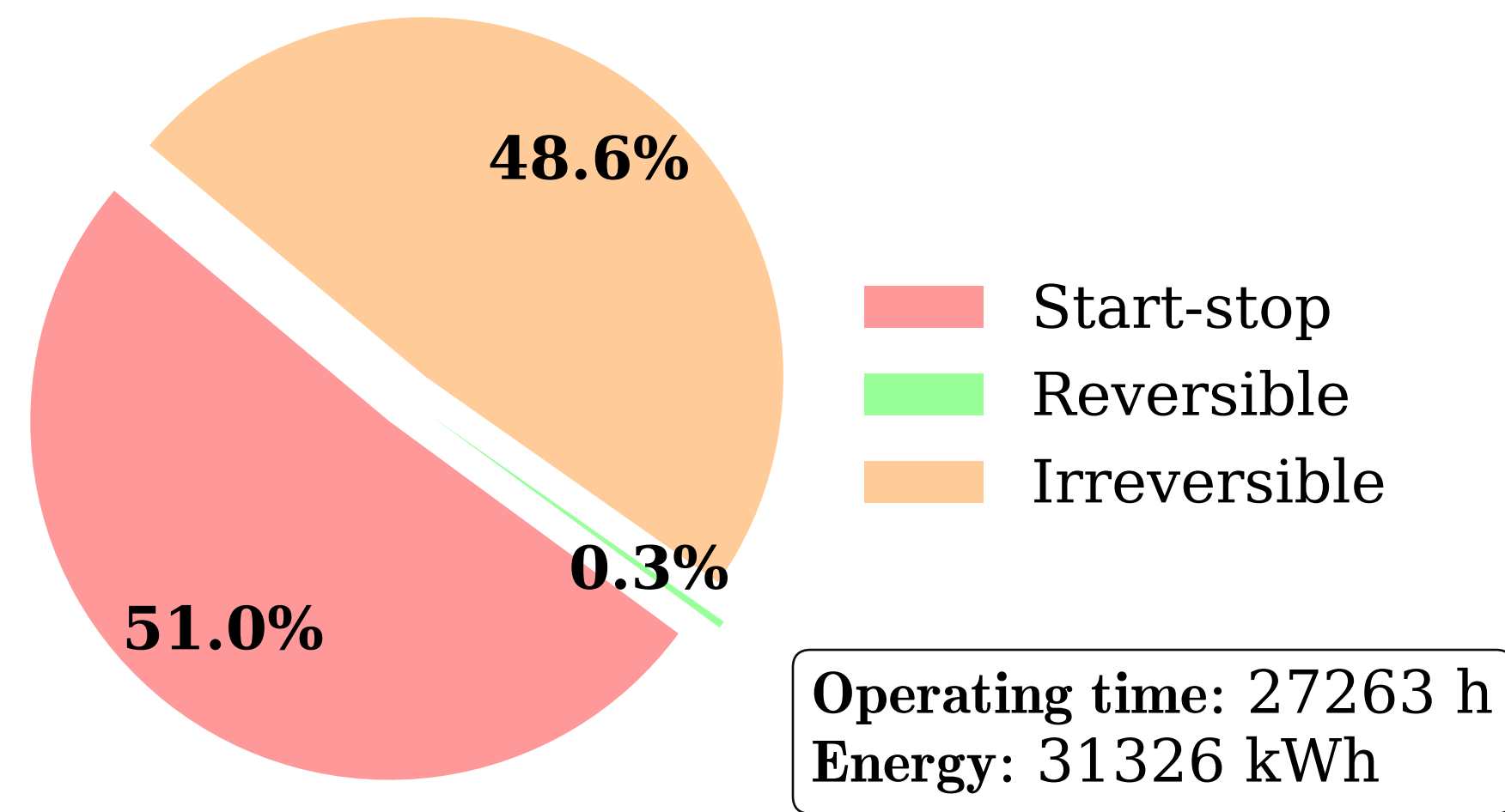
PEMFC Degradation
