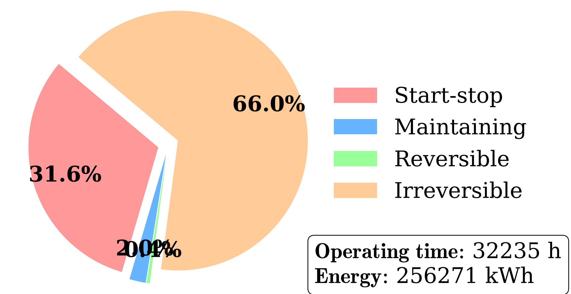
PEMWE Degradation
