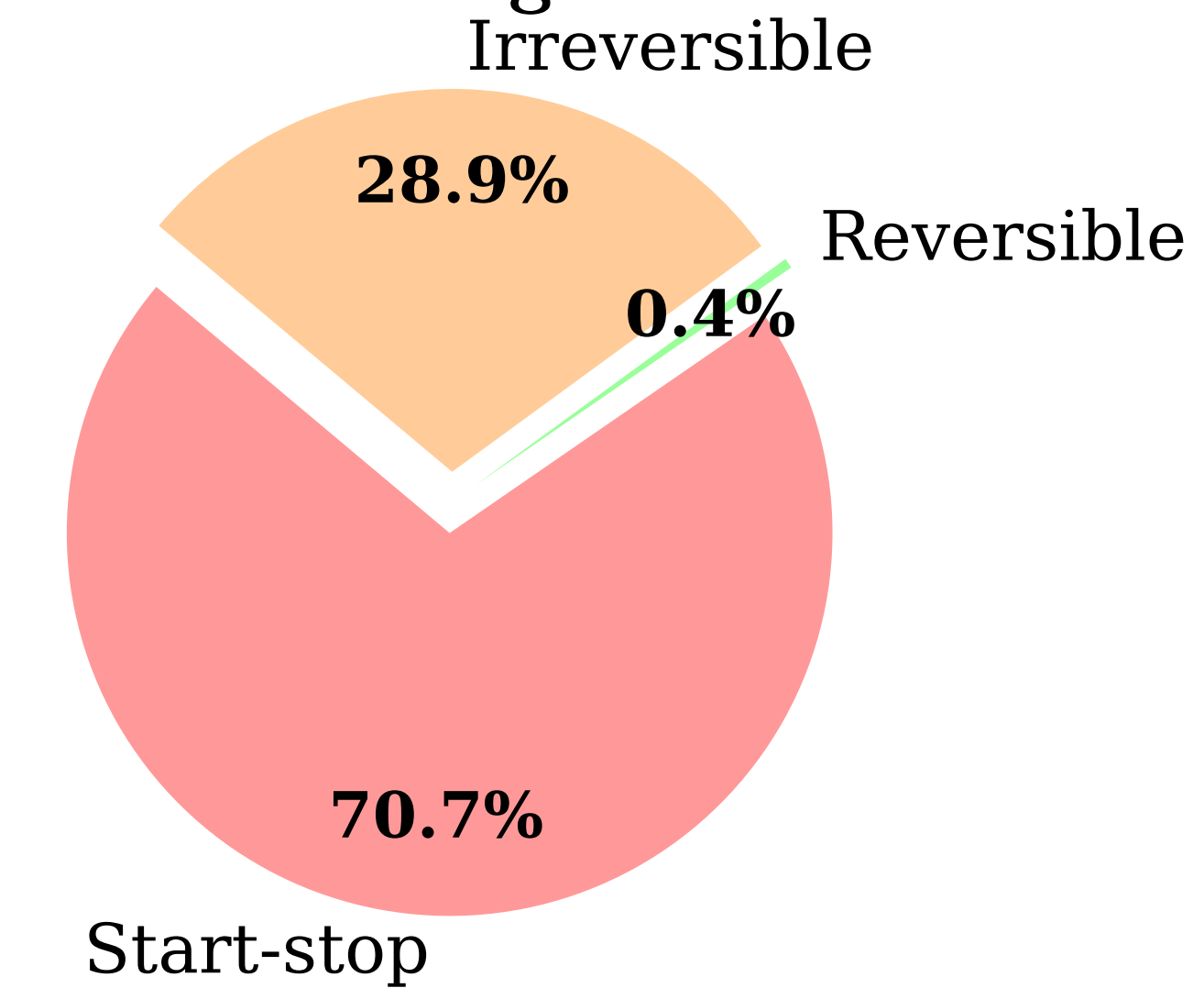
PEMWE Degradation
