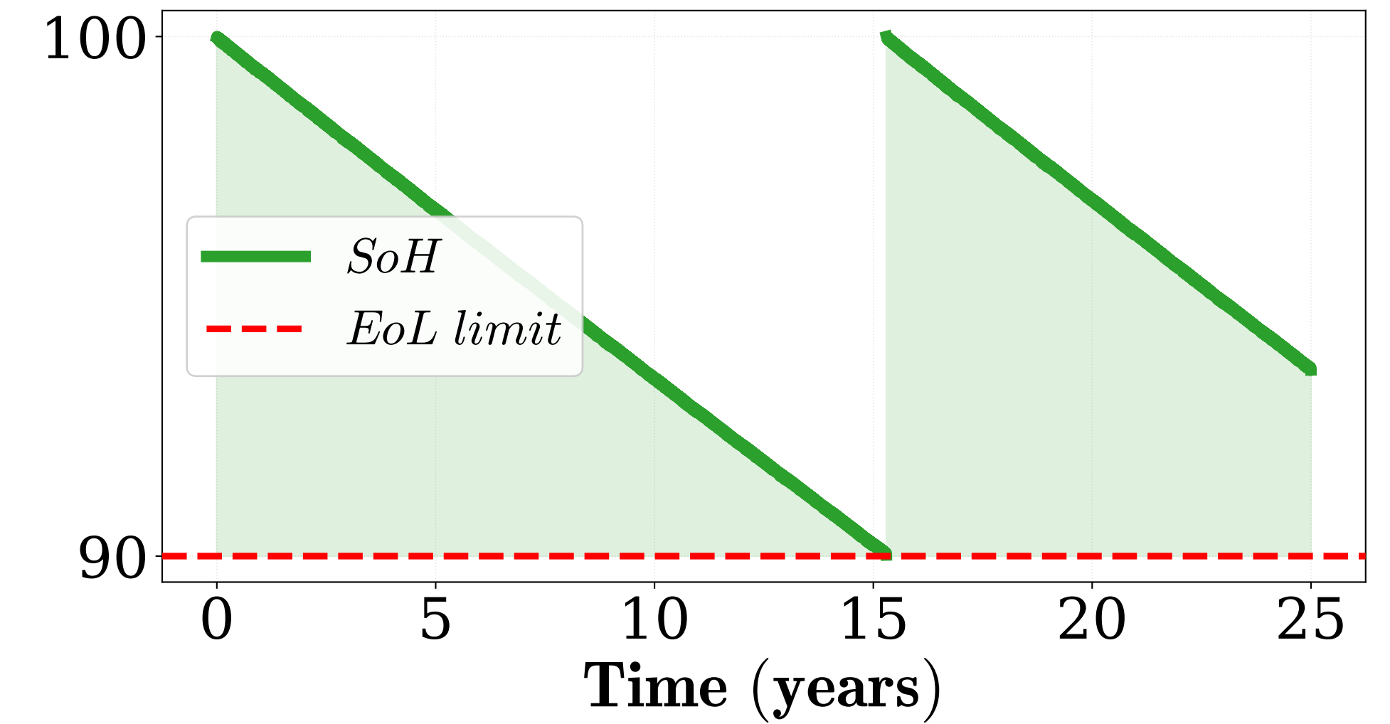
PEMWE Degradation
