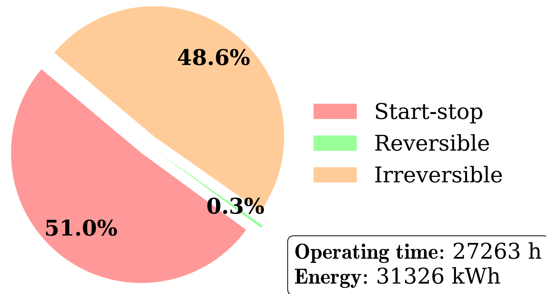
PEMFC Degradation
