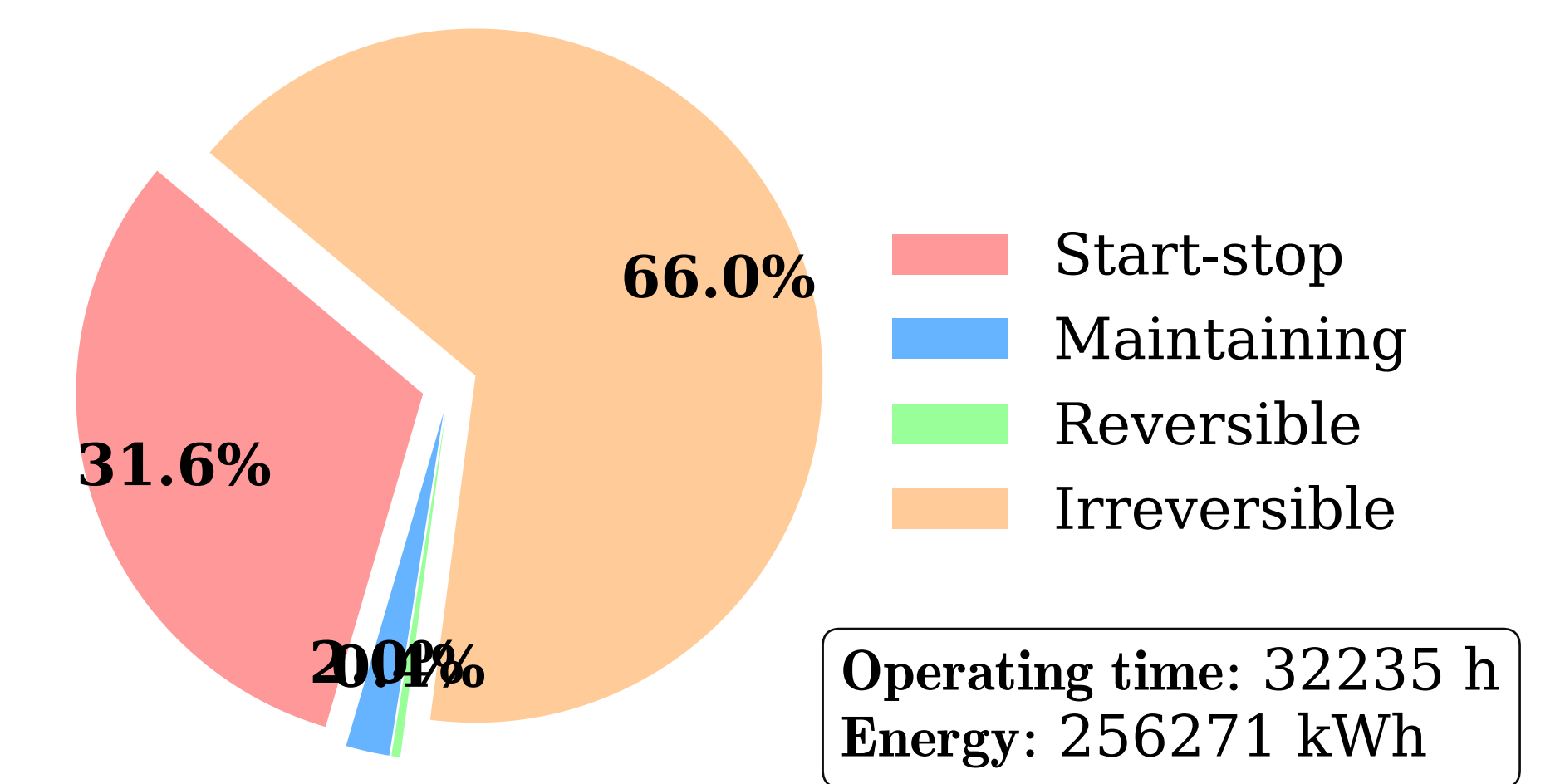
PEMWE Degradation
