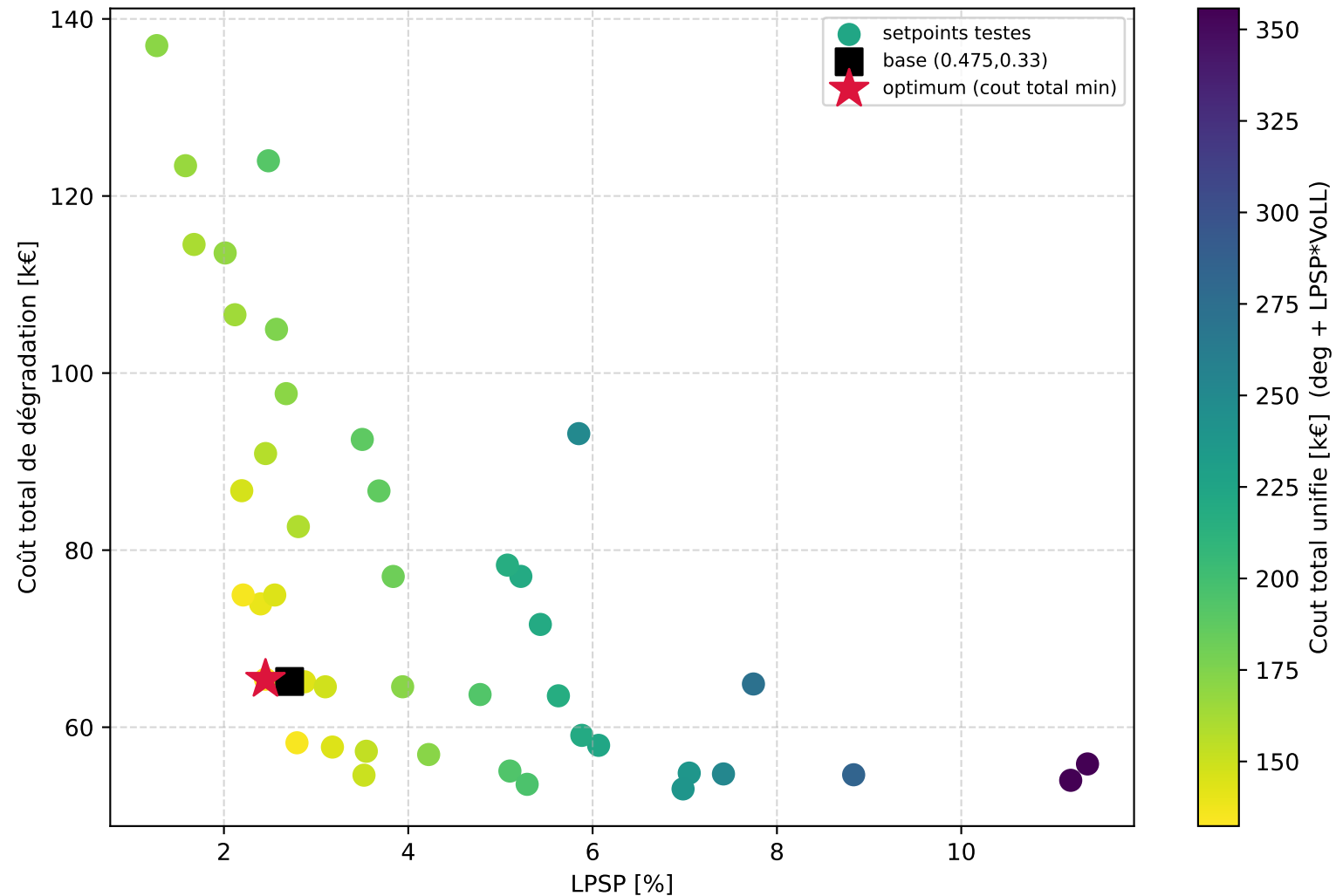
RB2 — setpoints minimisant le coût unifié (deg + LPSP financierisé VoLL) 25 ans, dimensionnement fixe
