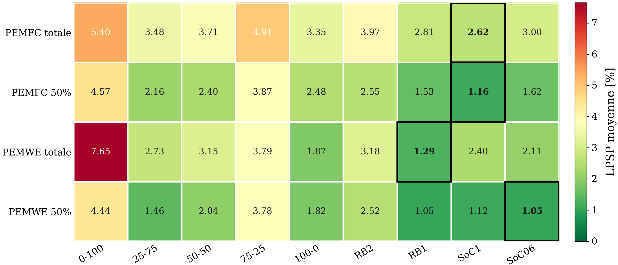
LPSP moyenne sous défaillance (la plus faible encadrée)
