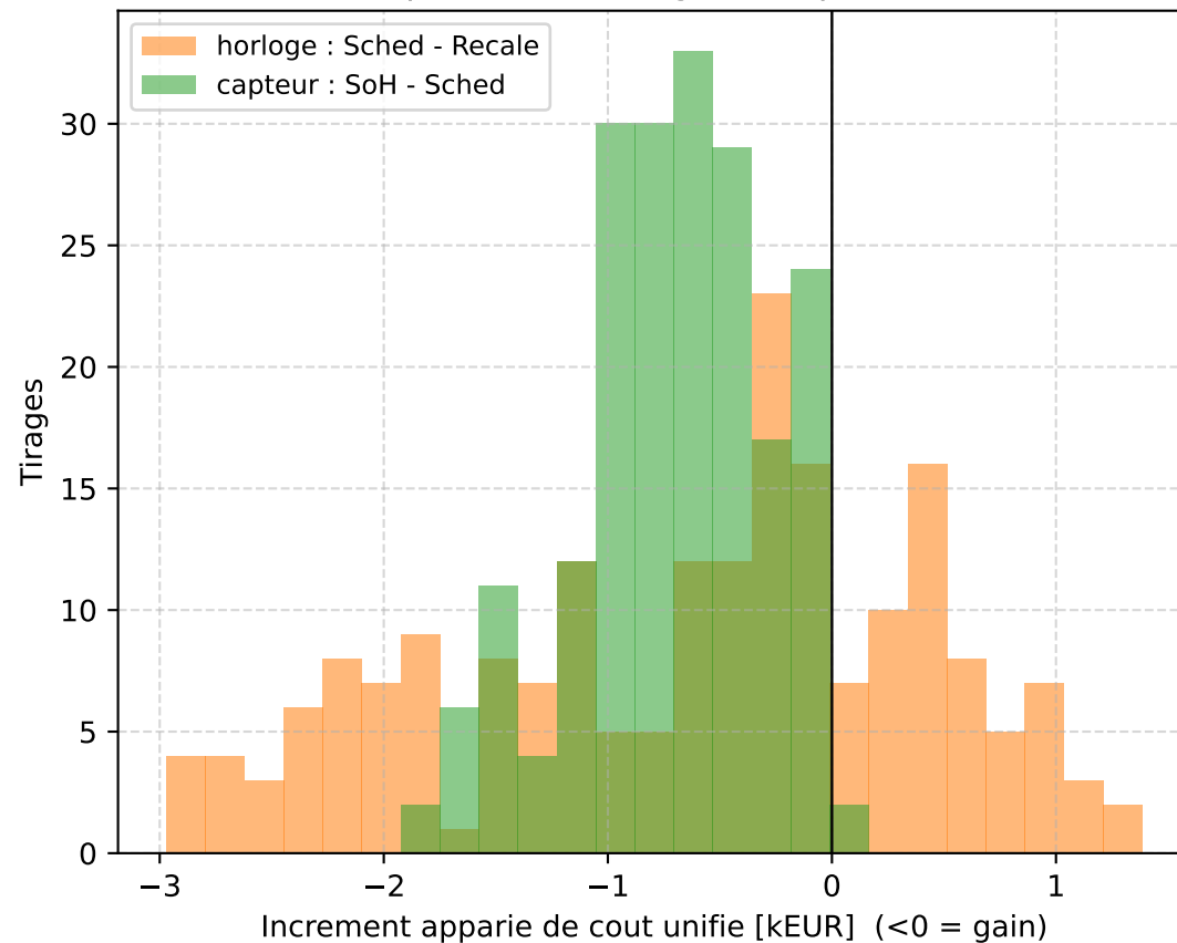
Decomposition : horloge vs capteur (CRN)
