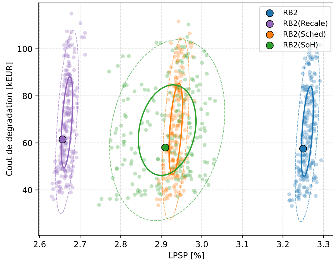
Incertitude du vieillissement : nuages + ellipses 1s/2s
