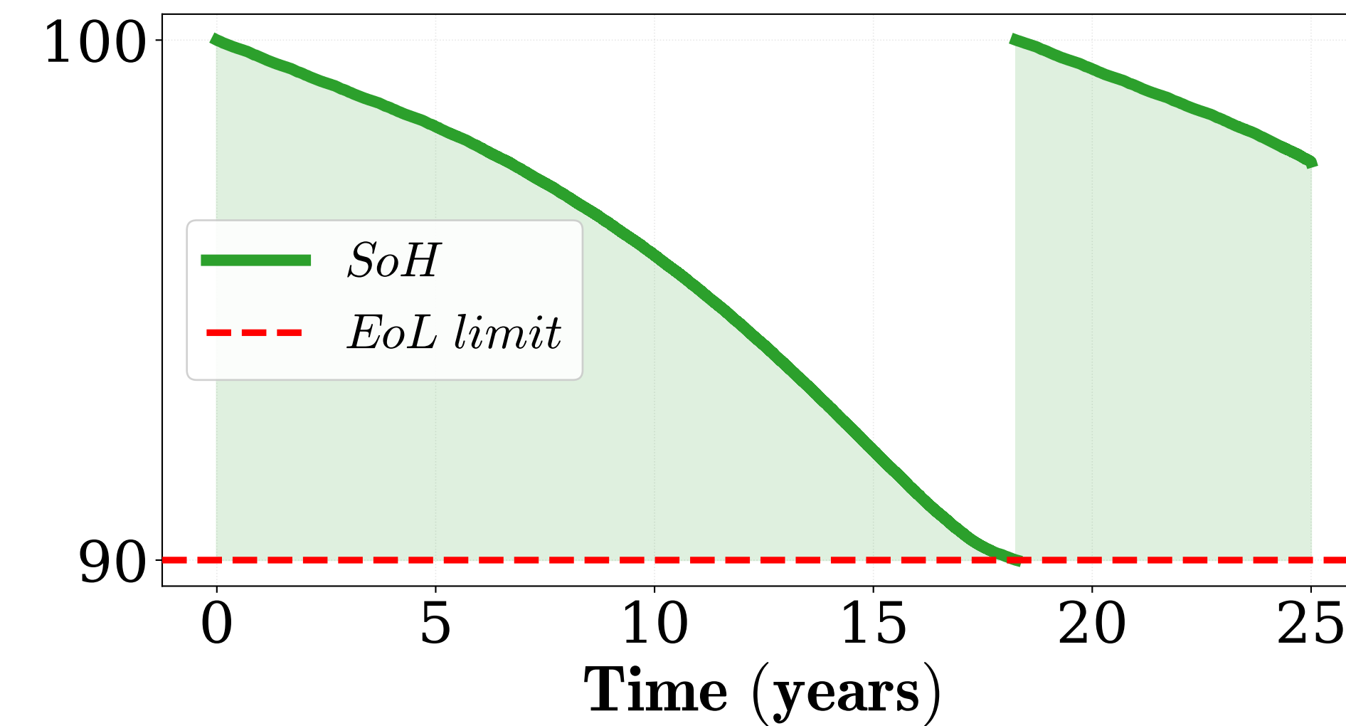
PEMWE Degradation
