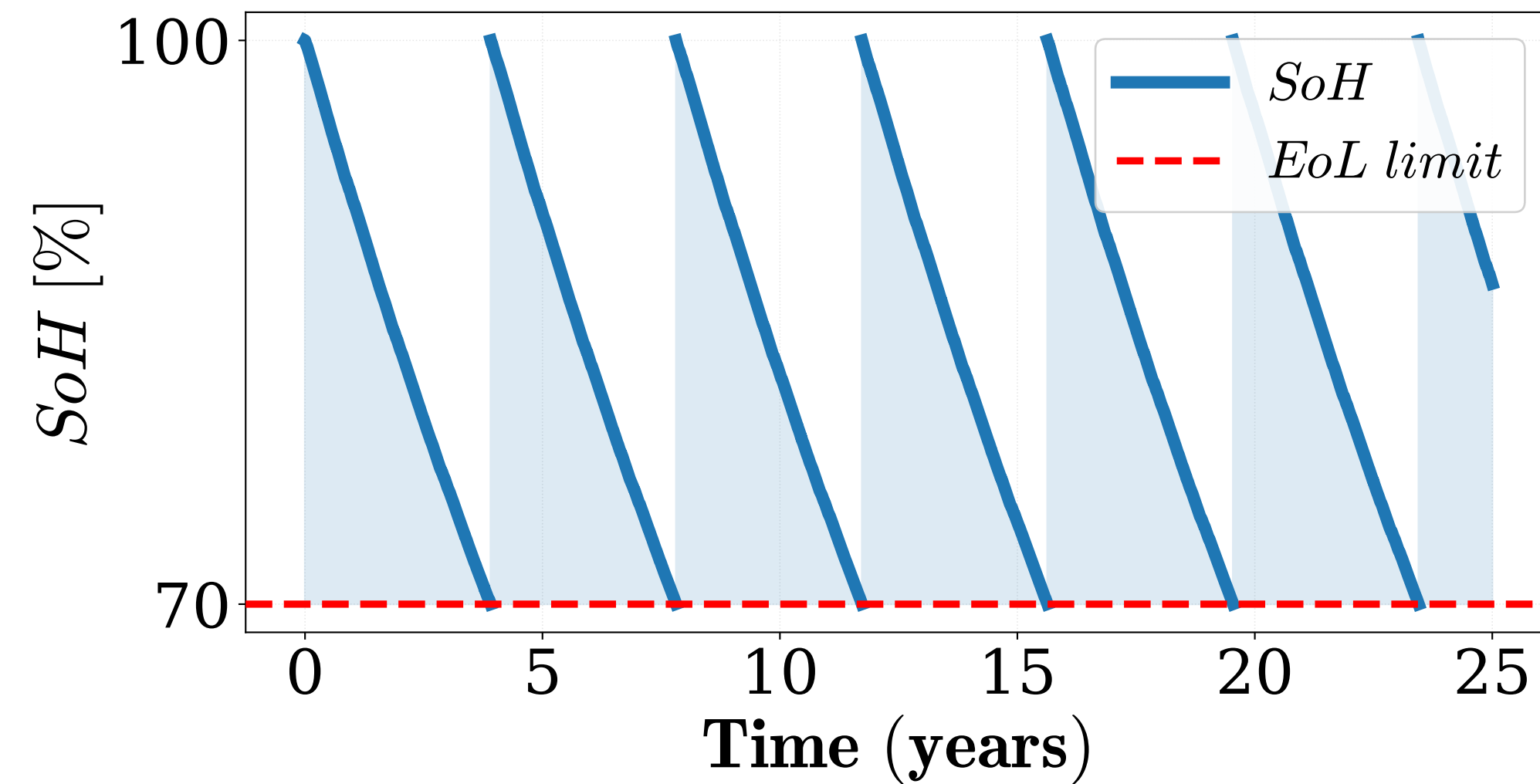
PEMFC Degradation
