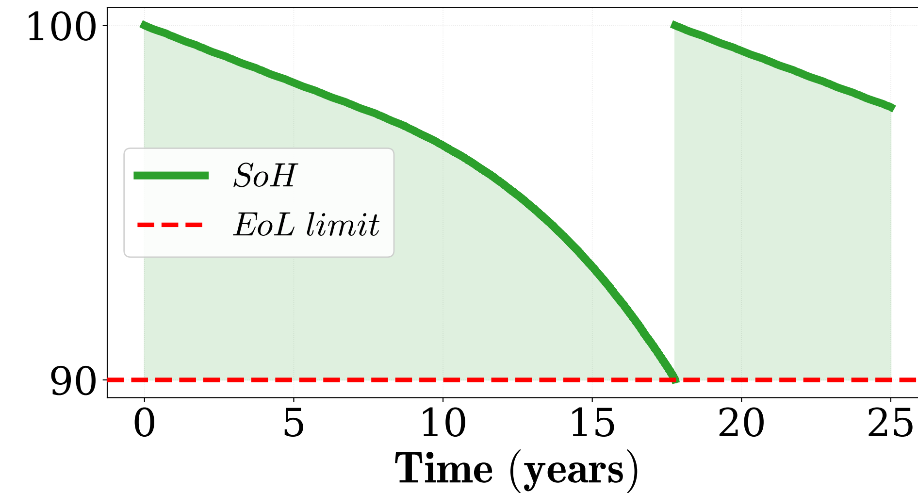
PEMWE Degradation
