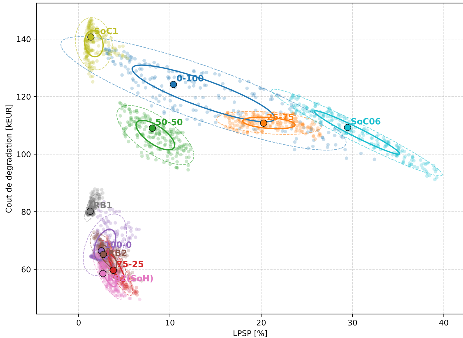
Robustesse du front de Pareto au dimensionnement (+/-20%)
