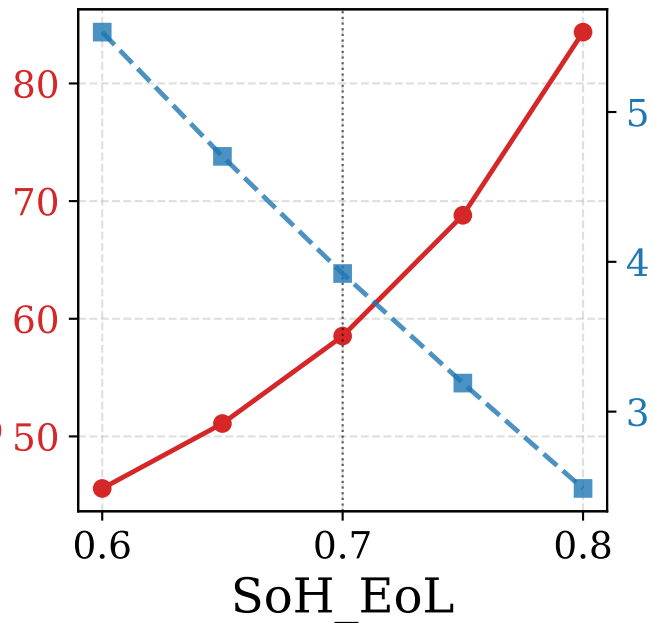
Batterie
