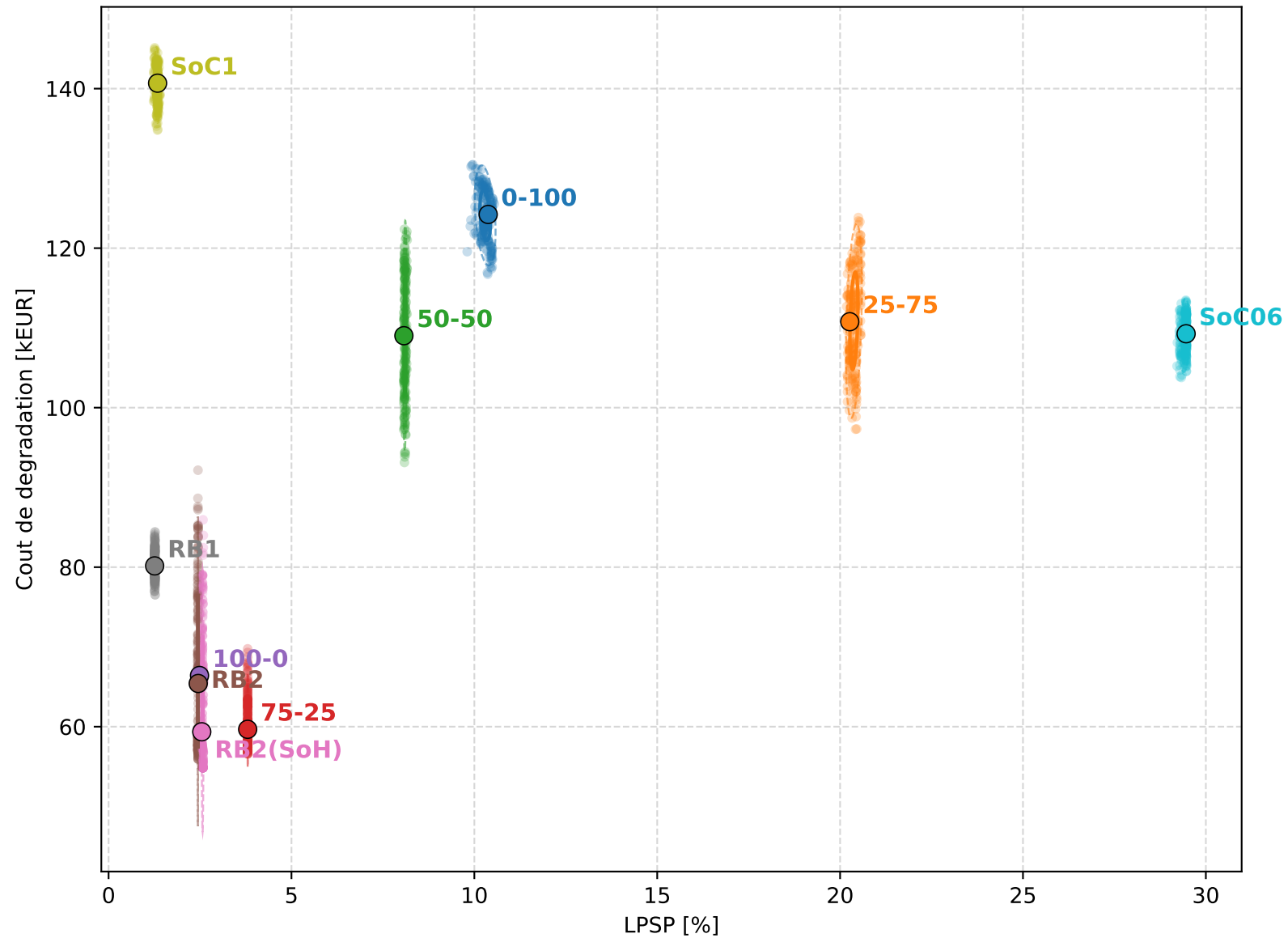
Robustesse du front de Pareto aux seuils de dégradation H2
