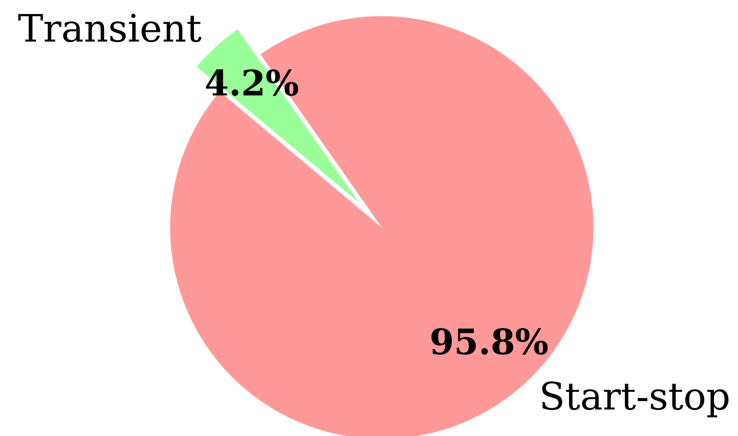
PEMFC Degradation
