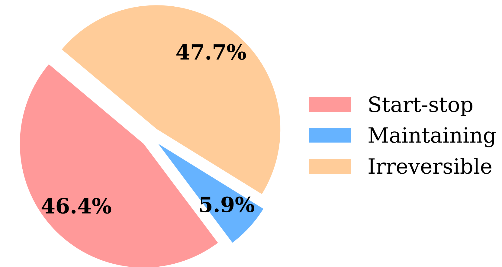
PEMWE Degradation
