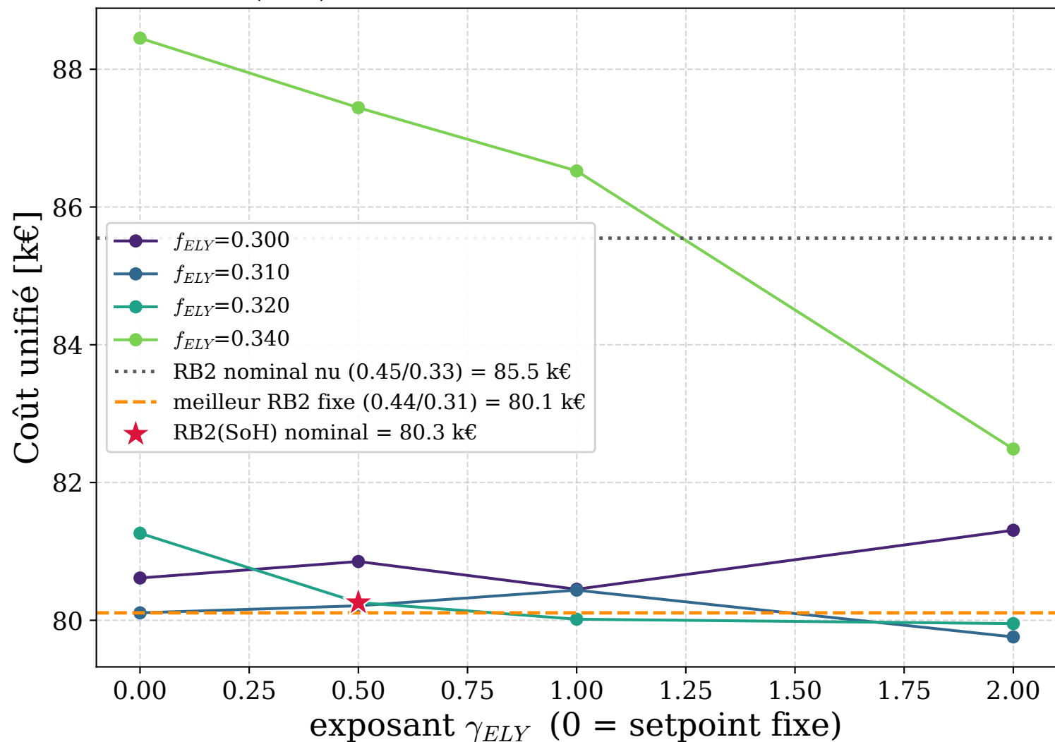
RB2(SoH) : coût unifié vs intensité de la modulation SoH
