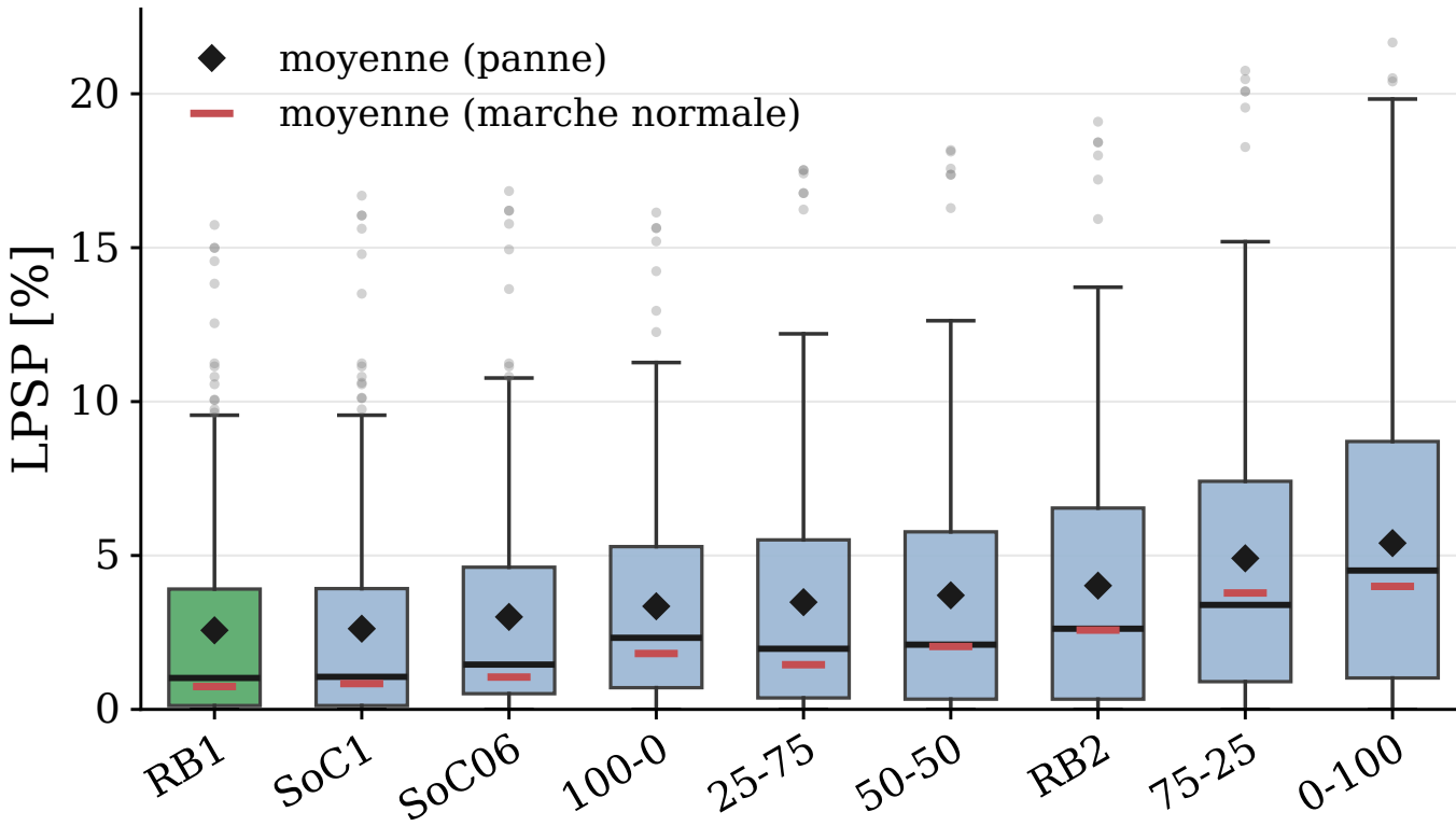
(a) PEMFC totale — meilleure : RB1
