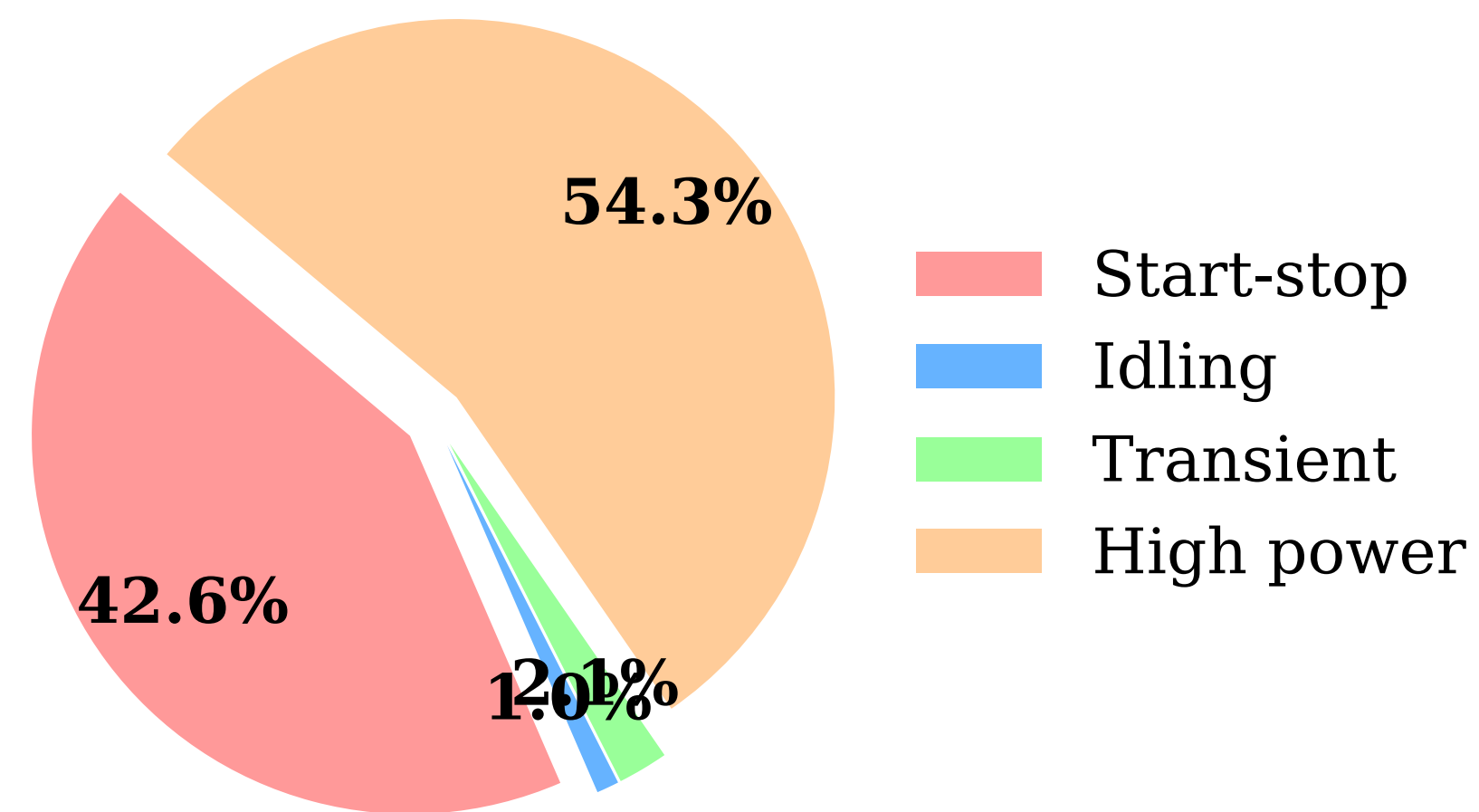
PEMFC Degradation
