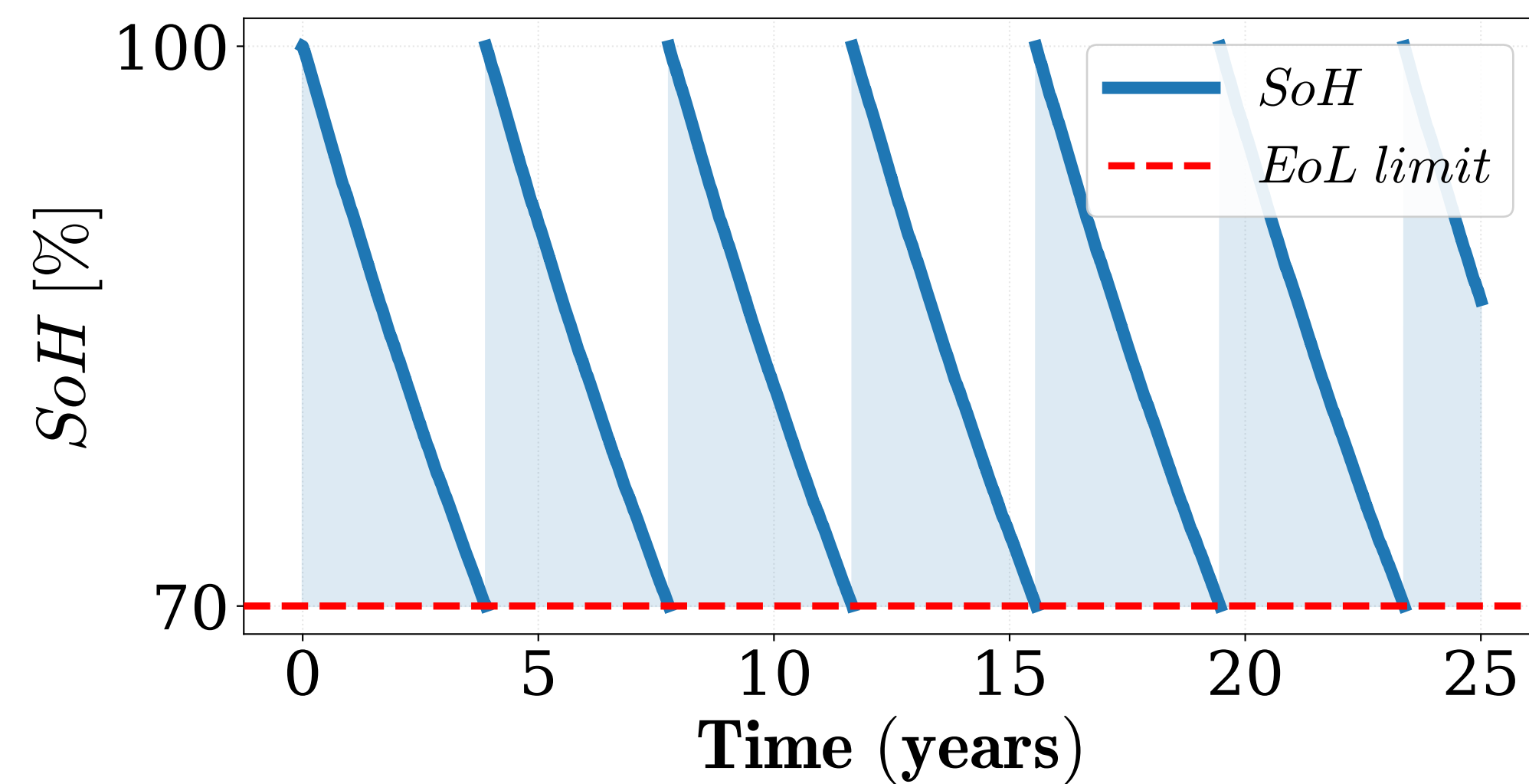
PEMFC Degradation
