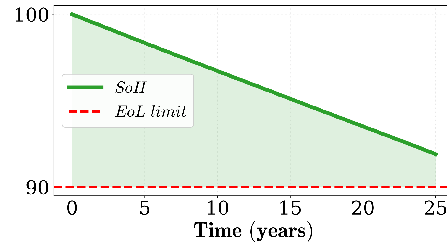
PEMWE Degradation
