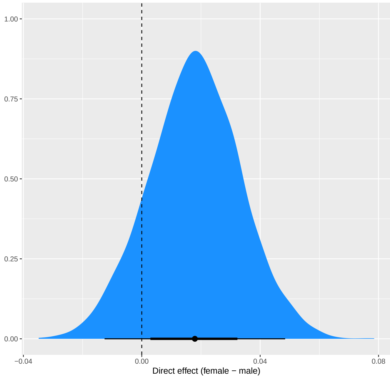
Posterior for the estimand
