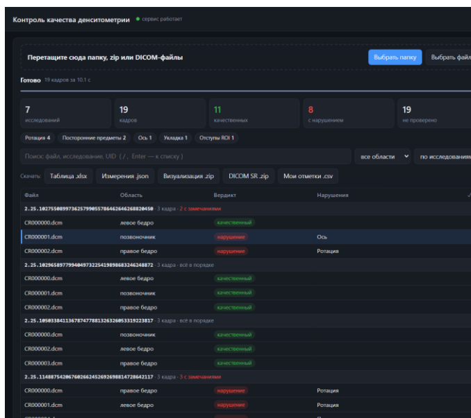
Веб-интерфейс: сводка по загруженному архиву и таблица по исследованиям (карточка со снимком не показана)
